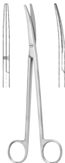
Ножницы для рассечения мягких тканей в глубоких полостях
