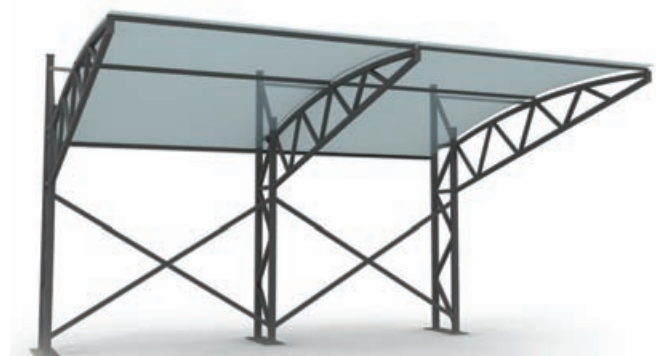
Консольный навес
