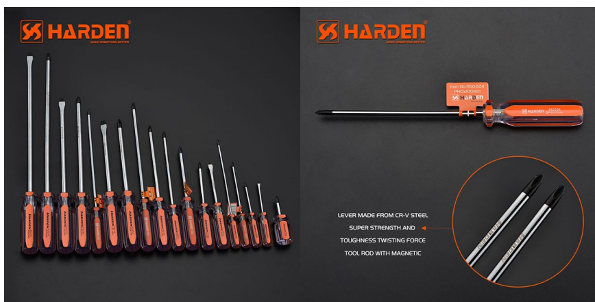
Отвертки с цветными рукоятками и намагниченными наконечником
