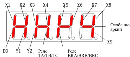
Рис. 6-29 Схема отображения текущего состояния статуса клемм
