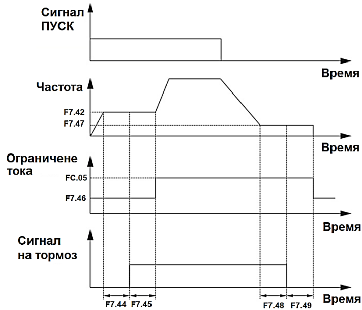
Рис. 6-23 Сигнал управления двигателя с электромеханическим тормозом
