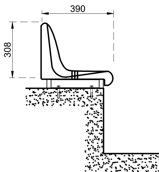
Вариант крепления стационарных сидений на металлоконструкции, установленных на бетонную поверхность гребенки
