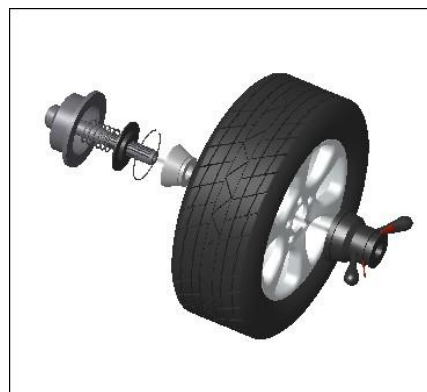
Вал- подходящий конус (вершиной наружу)
