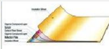
Нагревательная панель в разрезе
