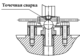
С-С вид в разрезе
