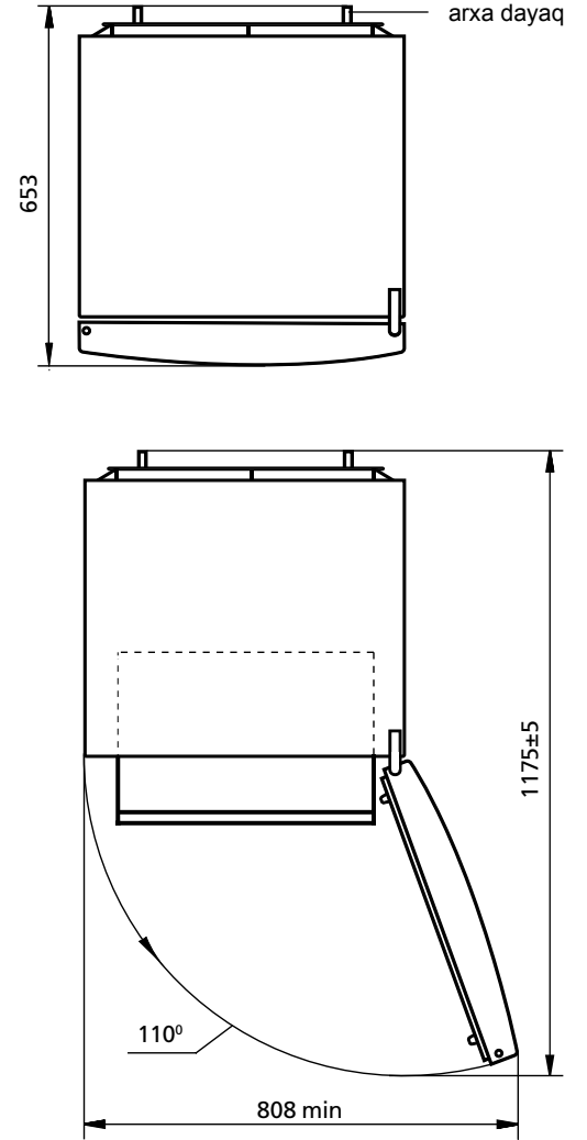
Şəkil 2 – Soyuducu (üstən görünüş)
