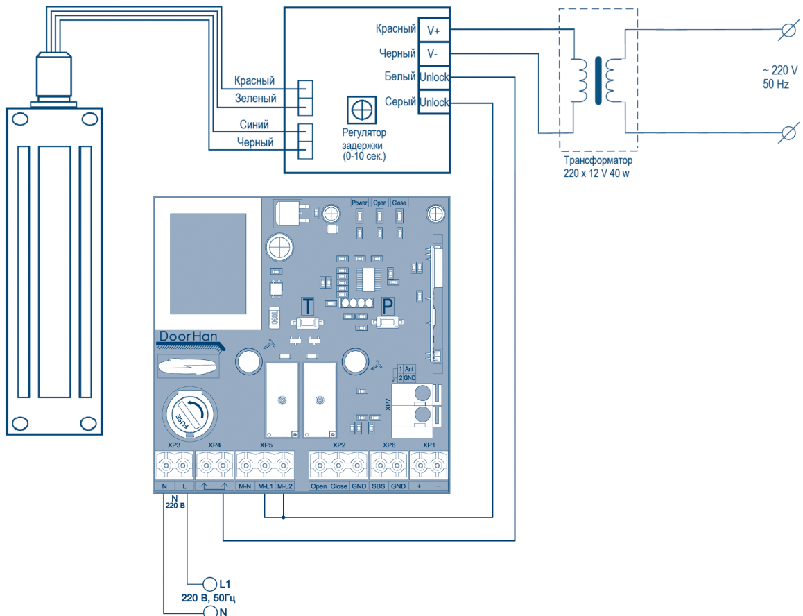
Рис. 4. Схема подключения электромагнитного замка
