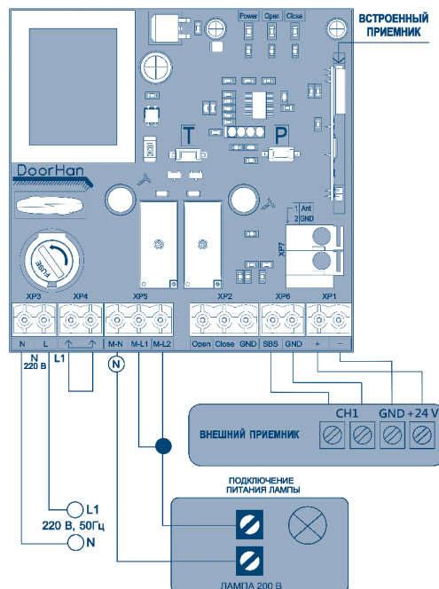
Рис. 2. Схема подключения освещения и внешнего радиуправления
