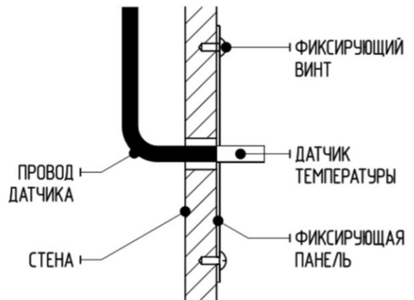
Рисунок 6. Установка датчика температуры
