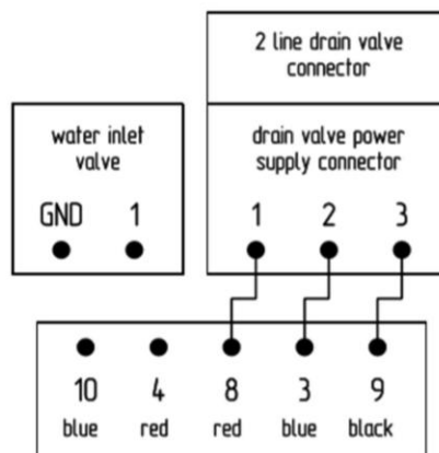
Рисунок 15. Описание последовательности VGA линии клапана подачи воды и сливного клапана
