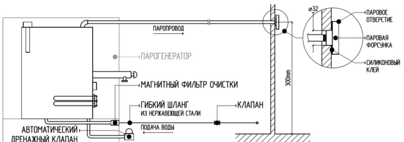
Рисунок 7. Схема подключения
