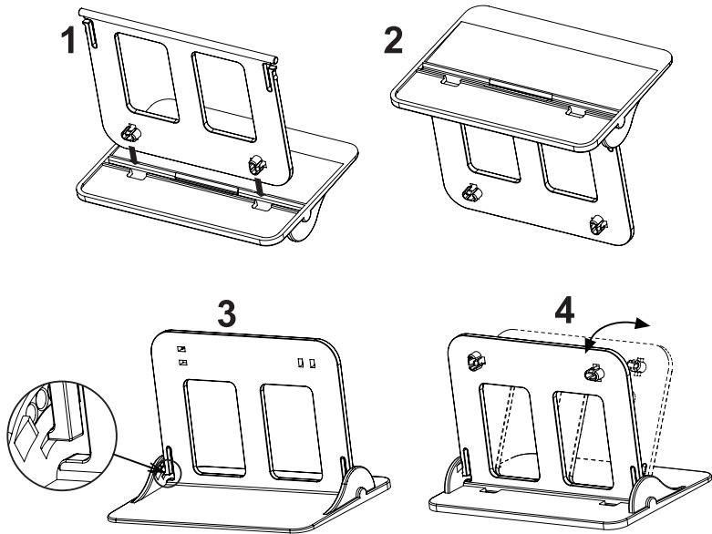
Рис. 7. Опора термостата
