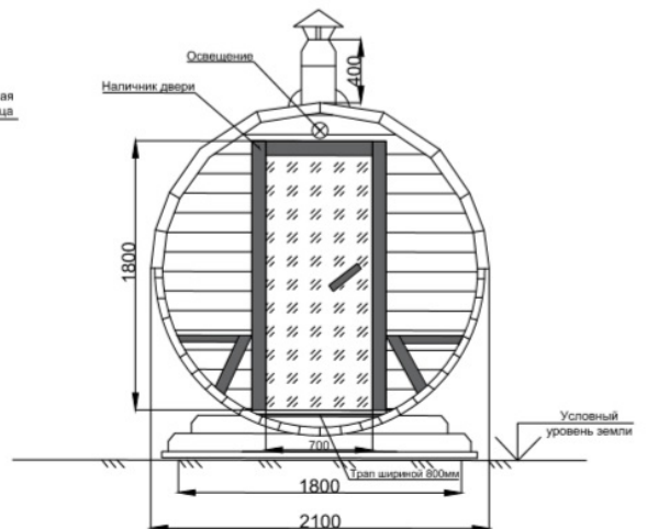
Парилка Вид от печи в сторону двери
