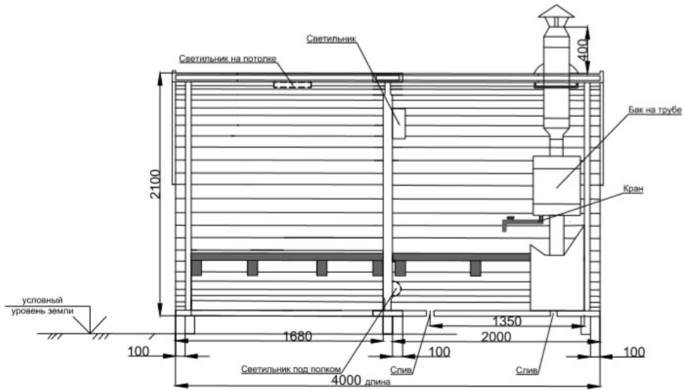
Парилка Вид от двери в сторону печи
