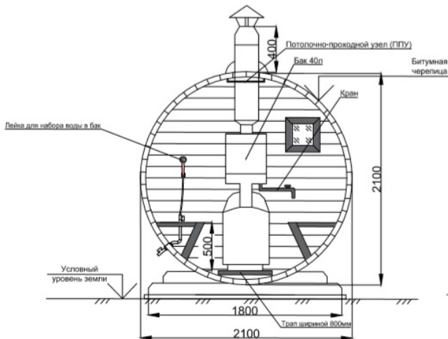
Парилка Вид от двери в сторону печи
