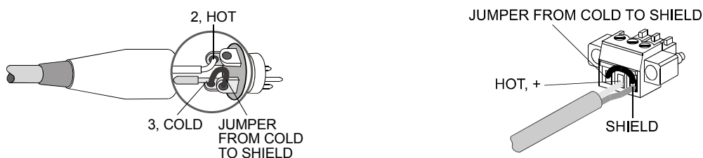
Illustration 2.11 : Connexion non-symétrisée de l'entrée
