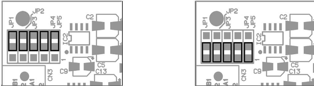
Abbildung 4.2: Jumperstellung in Pre-Fader-Betriebsart (links) und Post-Fader-Betriebsart (rechts)
