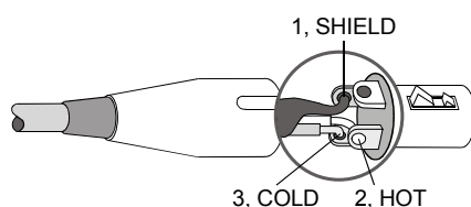
Illustration 2.12 : Connexion symétrisée de la sortie (Daisy-Chain)
