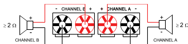
Abbildung 2.14: Lautsprecheranschluss in Betriebsart NORMAL an Anschlussklemmen
