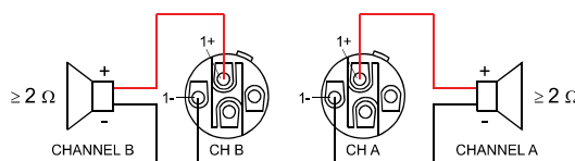
Abbildung 2.13: Lautsprecheranschluss in Betriebsart NORMAL an Speakon A und B
