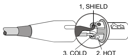
Abbildung 2.12: Symmetrische Beschaltung des Ausgangs (Daisy-Chain)
