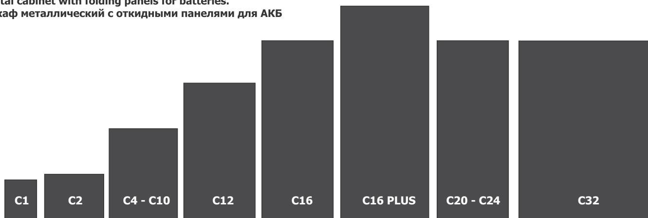
Aldyňgy körinis / Front view / Вид спереди
