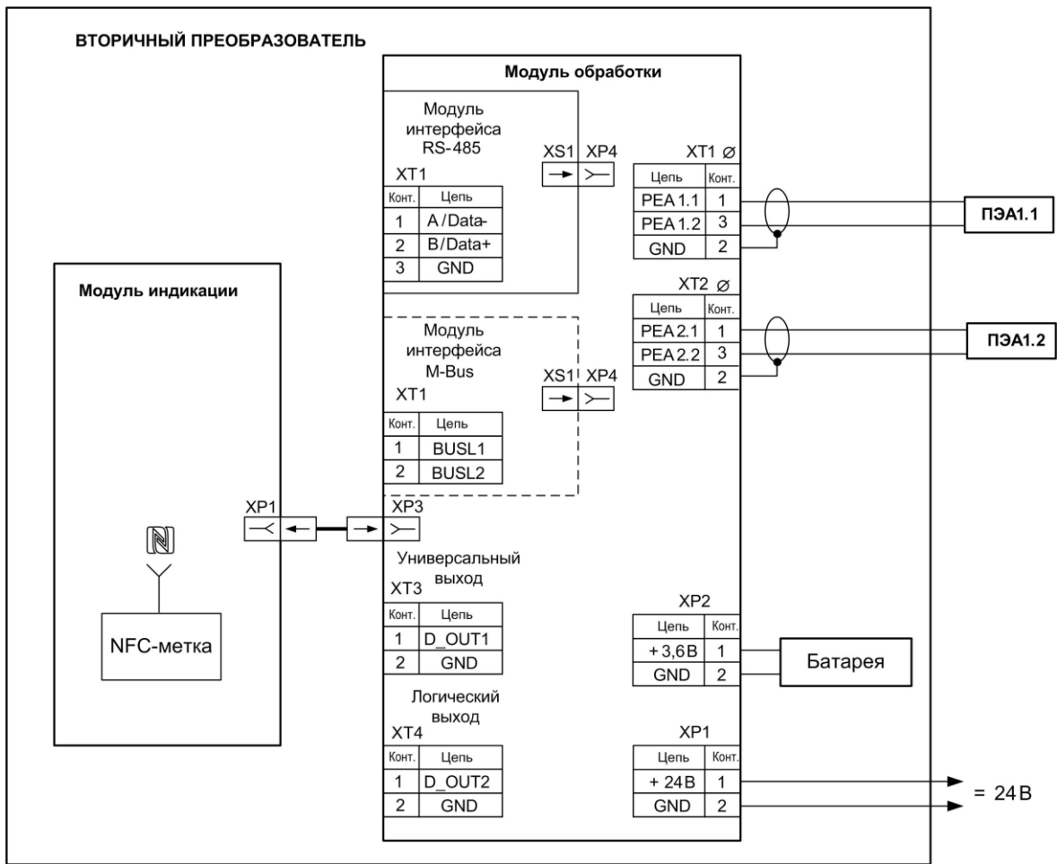
Рис.Б.1. Схема соединений расходомера УПСВ-311.
