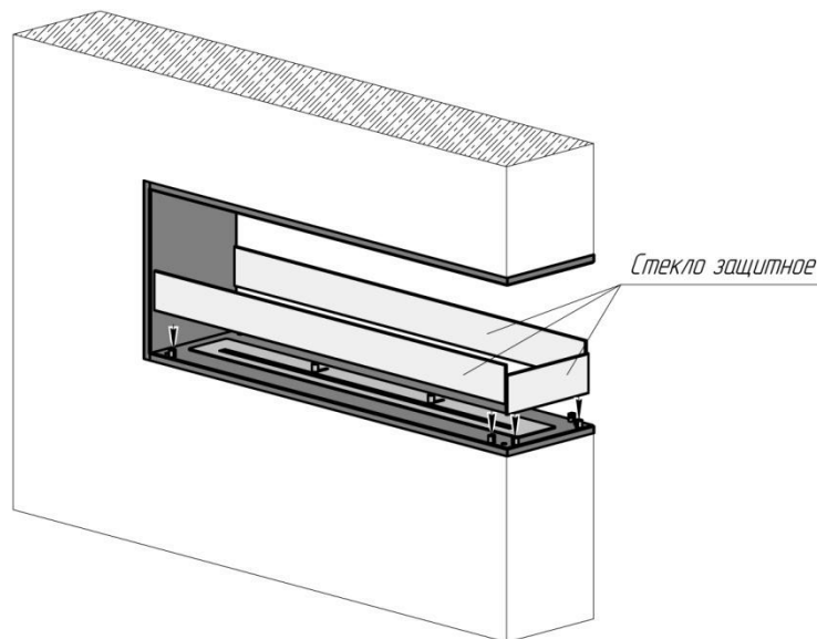
Рис.4 Установить защитное стекло
