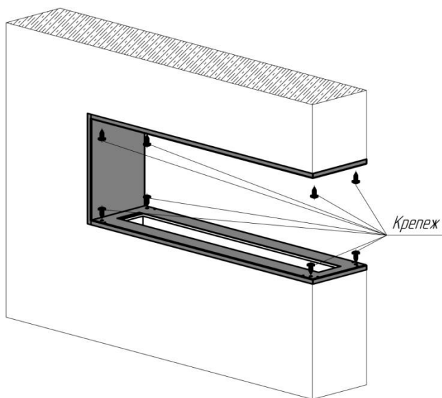
Рис.2 Закрепить биокамин в нише сверху и снизу
