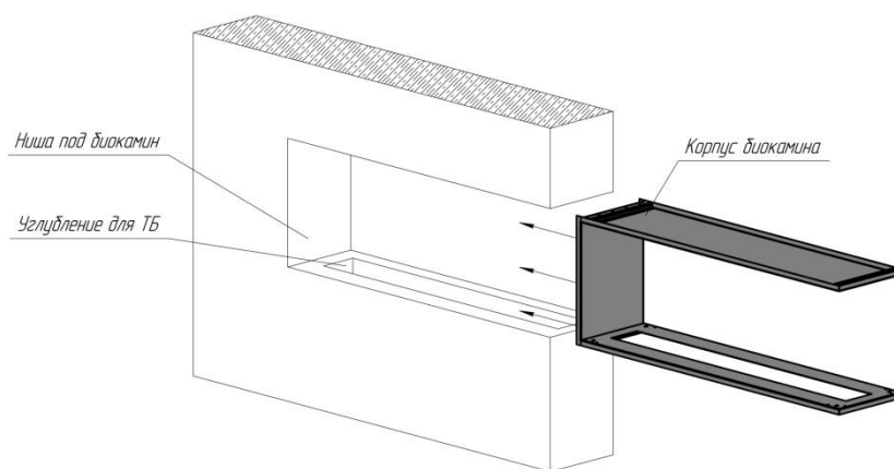
Рис.1 Поместить корпус биокамина в подготовленную нишу.
