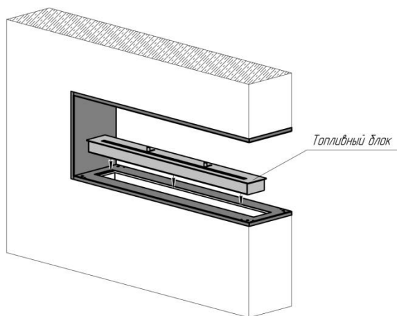
Рис.3 Установить топливный блок
