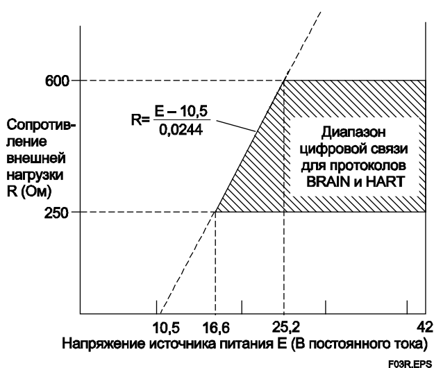
Рис. 2. Взаимосвязь между напряжением источника питания и сопротивлением внешней нагрузки Напряжение питания "◇"
