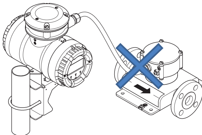
Рис. 11. Положение при установке, которого необходимо избегать: Расходомер в наклонном положении
