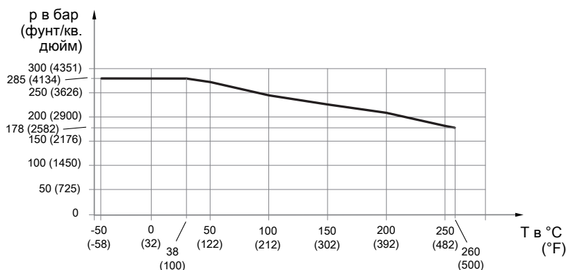
Рис. 20. Допустимое давление технологического процесса в зависимости от температуры в месте технологического присоединения
