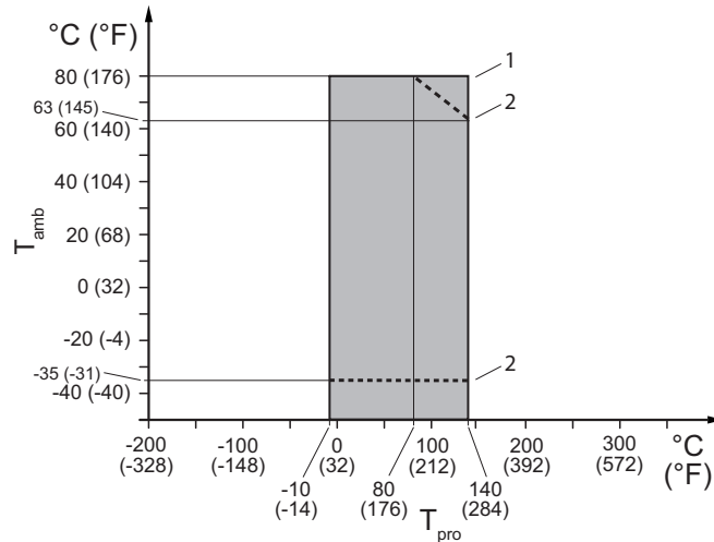
Рис. 23. Допустимая температура рабочей среды и окружающей среды, разнесенное исполнение, для типа присоединения к технологическому процессу HS4 и HS8
