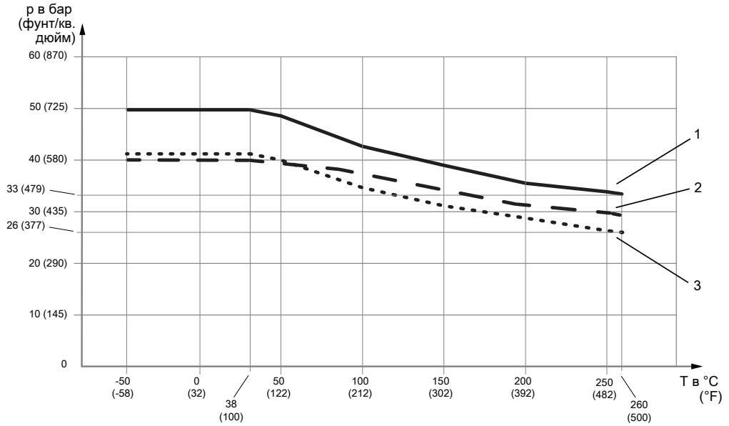
Рис. 13. Допустимое давление технологического процесса в зависимости от температуры в месте технологического присоединения
