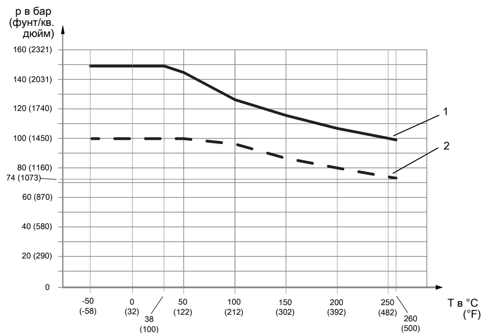
Рис. 15. Допустимое давление технологического процесса в зависимости от температуры в месте технологического присоединения
