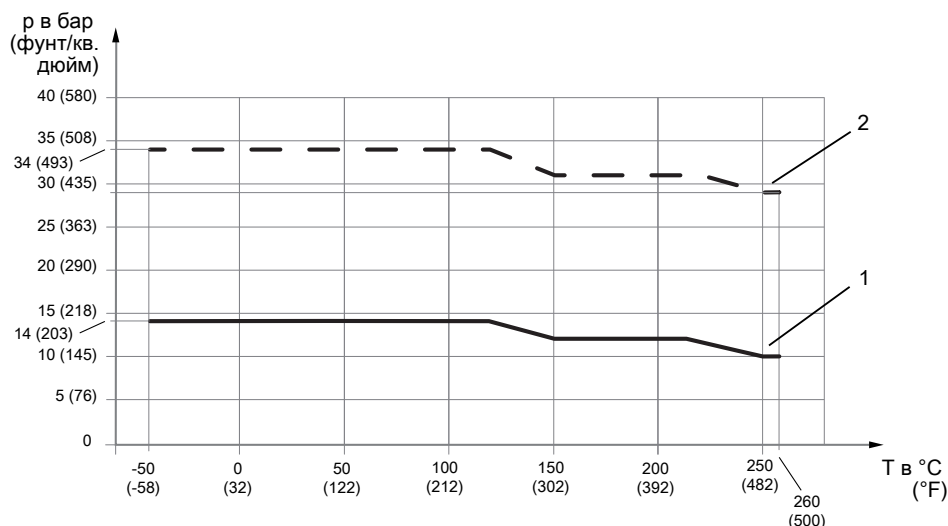
Рис. 17. Допустимое давление технологического процесса в зависимости от температуры в месте технологического присоединения
