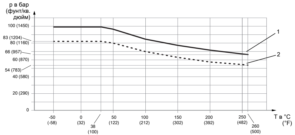
Рис. 14. Допустимое давление технологического процесса в зависимости от температуры в месте технологического присоединения
