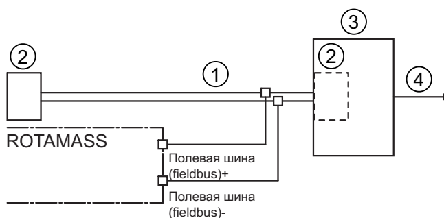
Рис. 47. Соединение PROFIBUS PA
