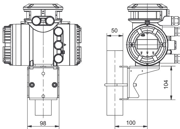
Рис. 30. Размеры измерительного преобразователя в мм, прикреплен к монтажному кронштейну.
