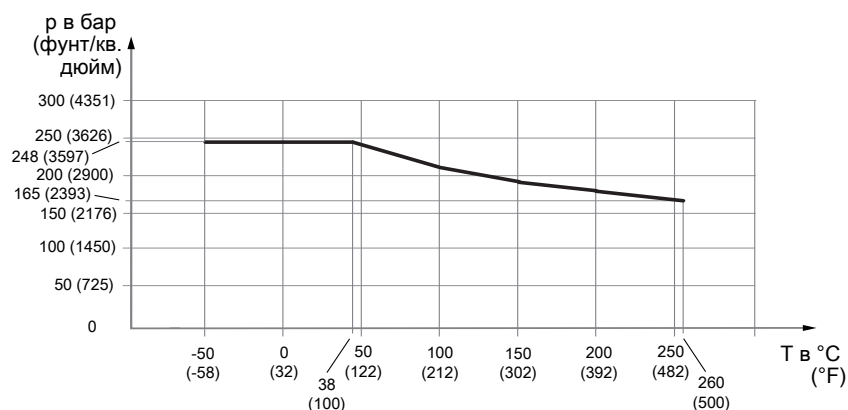
Рис. 16. Допустимое давление технологического процесса в зависимости от температуры в месте технологического присоединения
