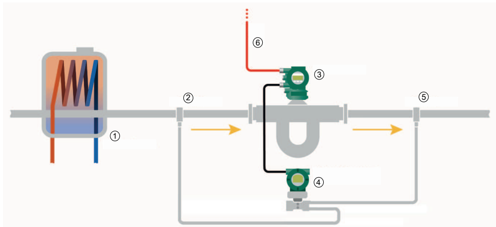
Рис. 52. Размещение точек измерения давления
