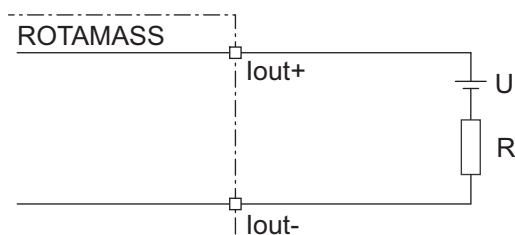
Рис. 33. Соединение пассивного токового выхода I_{out}
