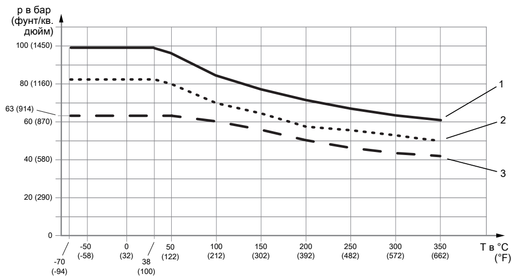
Рис. 15. Допустимое давление технологического процесса в зависимости от температуры в месте технологического присоединения
