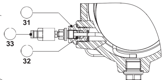
HVV - Ручной вентиляционный клапан
