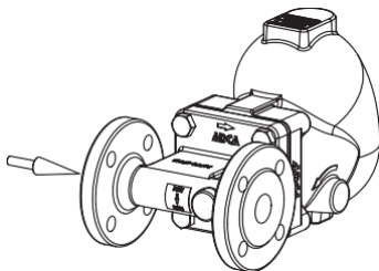
Установка на горизонтальном трубопроводе, направление потока слева направо ( IL ).
