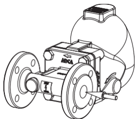
Установка на горизонтальном трубопроводе, направление потока справа налево ( IR ).
