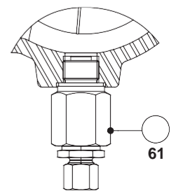
AFZ - Устройство защиты от заморозания (Автоматический)
