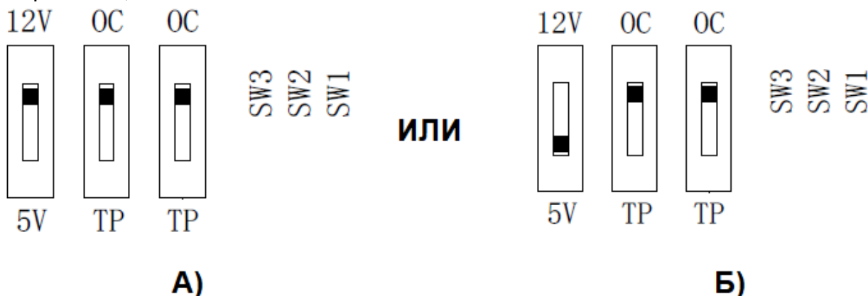
Рисунок 7-3 Коллектор открытого типа, двухтактный датчик, выбор DIP-переключателя. Изображение А выбор питания 12 вольт, изображение Б выбор питания 5 вольт
