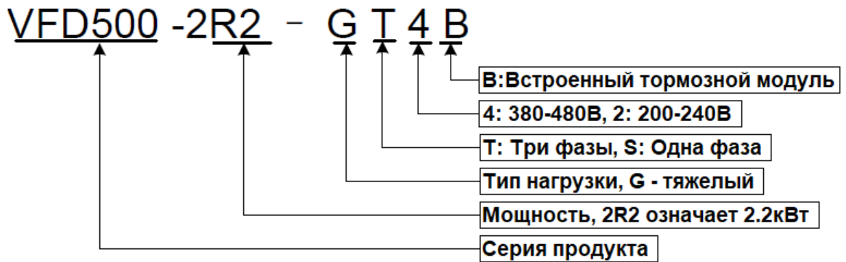
Рисунок 2-1 Условные обозначения
