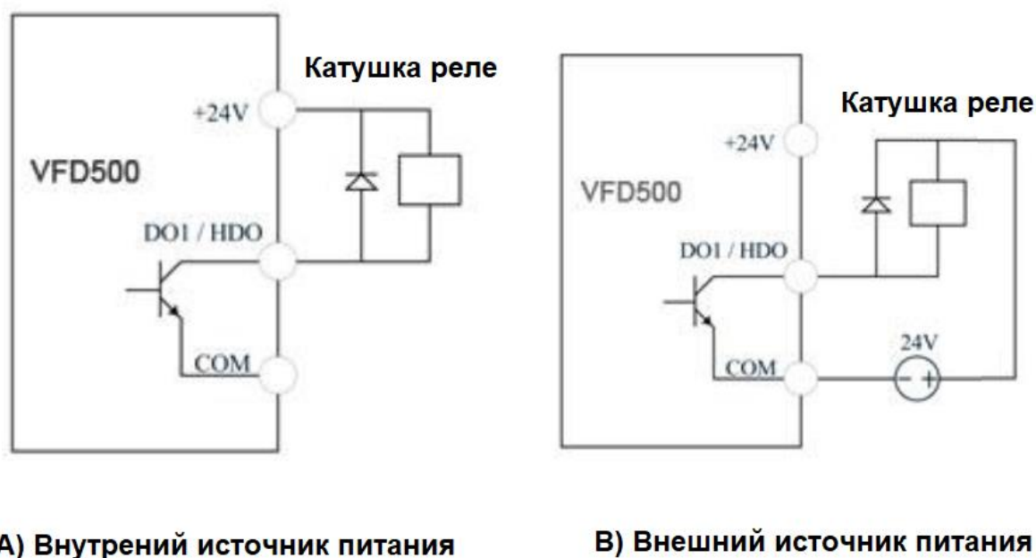
Рисунок 3-22 Подключение цифрового выхода
