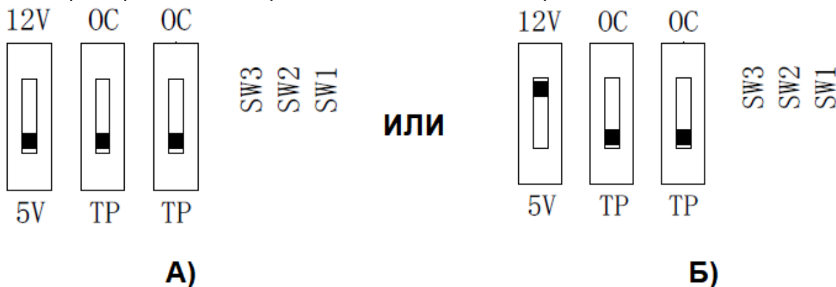
Рисунок 7-5 Коллектор открытого типа, дифференциальный энкодер, выбор DIP-переключателя. Изображение А выбор питания 5 вольт, изображение Б выбор питания 12 вольт
