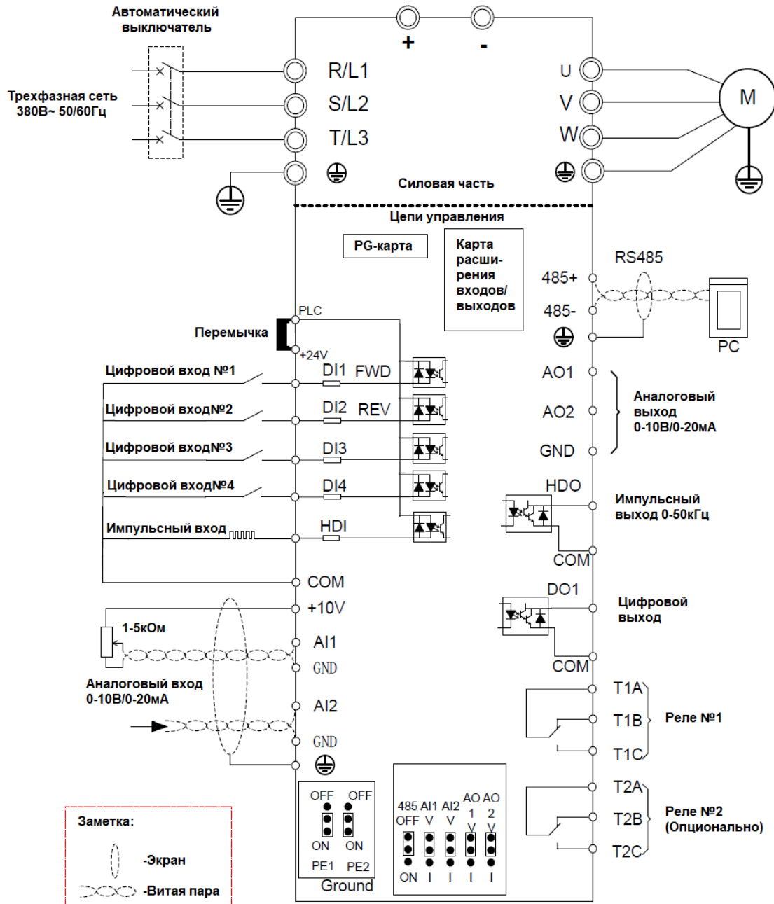
Рисунок 3-13 Схема подключений ПЧ серии VFD500 типоразмеров E и выше
