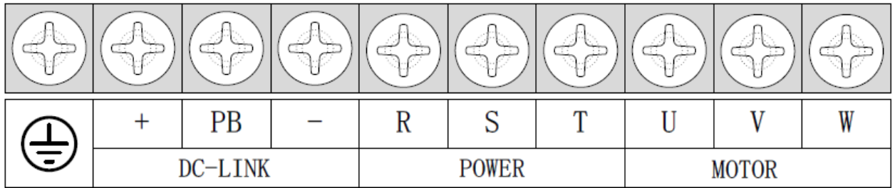
Рисунок 3-14 Подключение силовых клемм для ПЧ типоразмеров А-С
