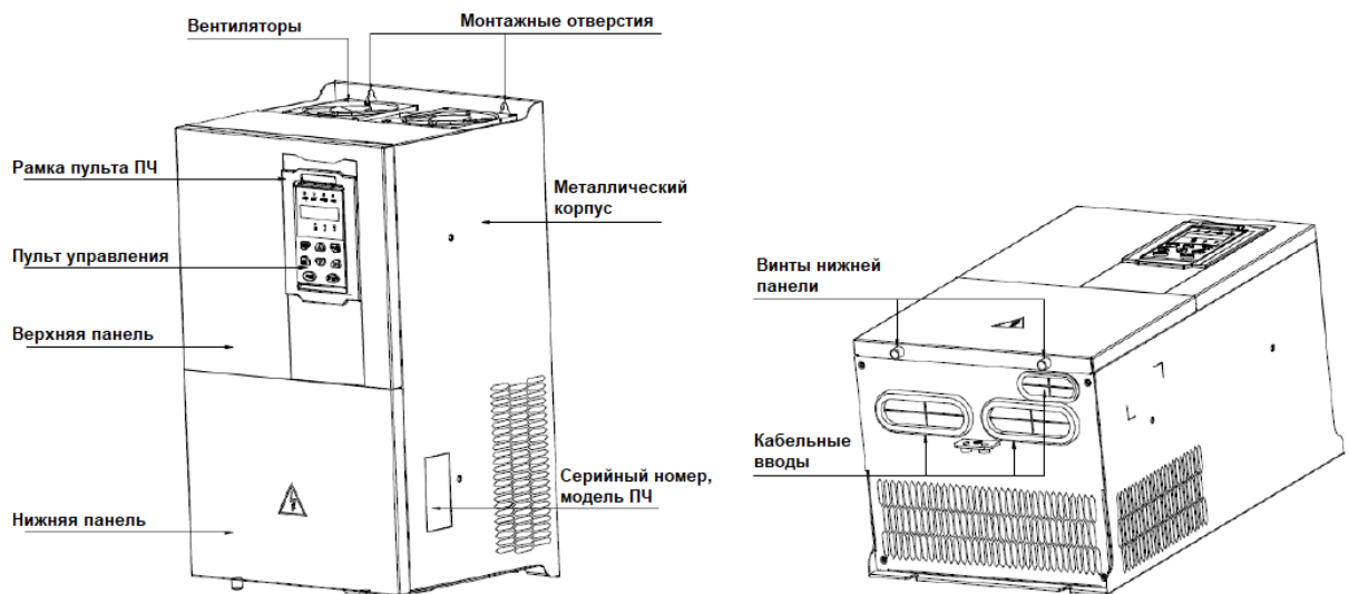
Рисунок 3-2 VFD500 металлический корпус
