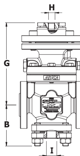
Рис. 3 - Клапан с крышкой для работы на сжатом воздухе
