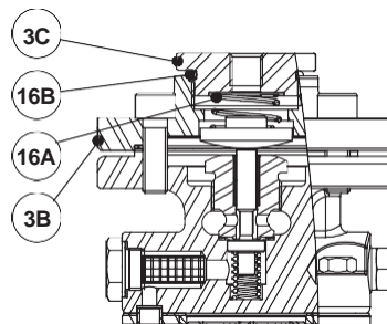
Купольная крышка для работы на сжатом воздухе
