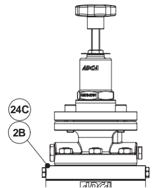
Переходный фланец (только DN 50)
