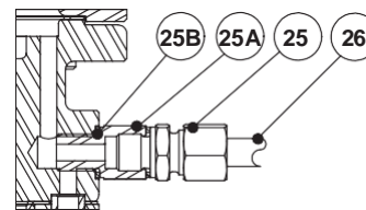
Стандартное исполнение Подсоединения внешней трубы отбора импульса давления
