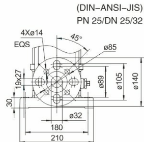
DIN фланец(LVS)
