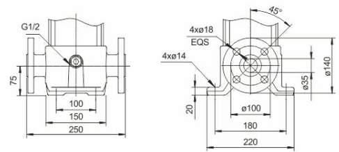
DIN фланец(LVR)
