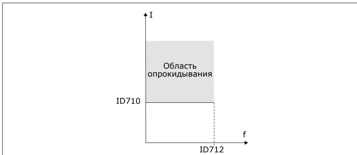
Рис. 68: Настройки характеристик опрокидывания.
