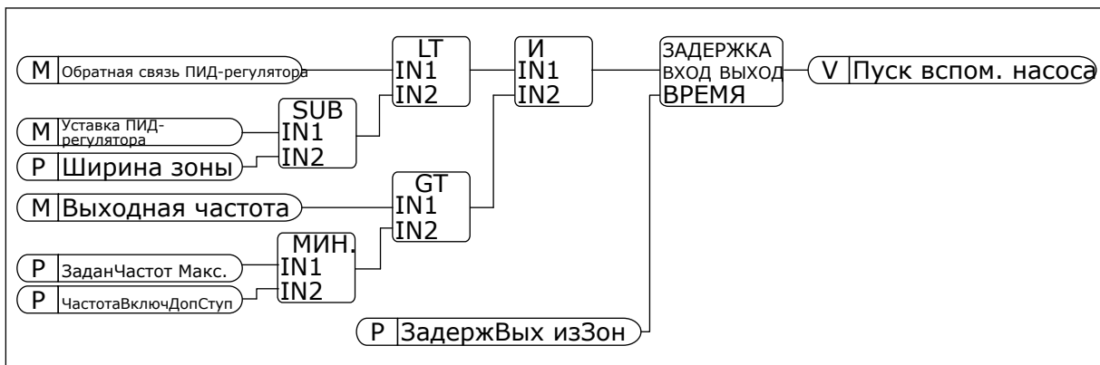
Рис. 101: Частота включения доп. ступени
