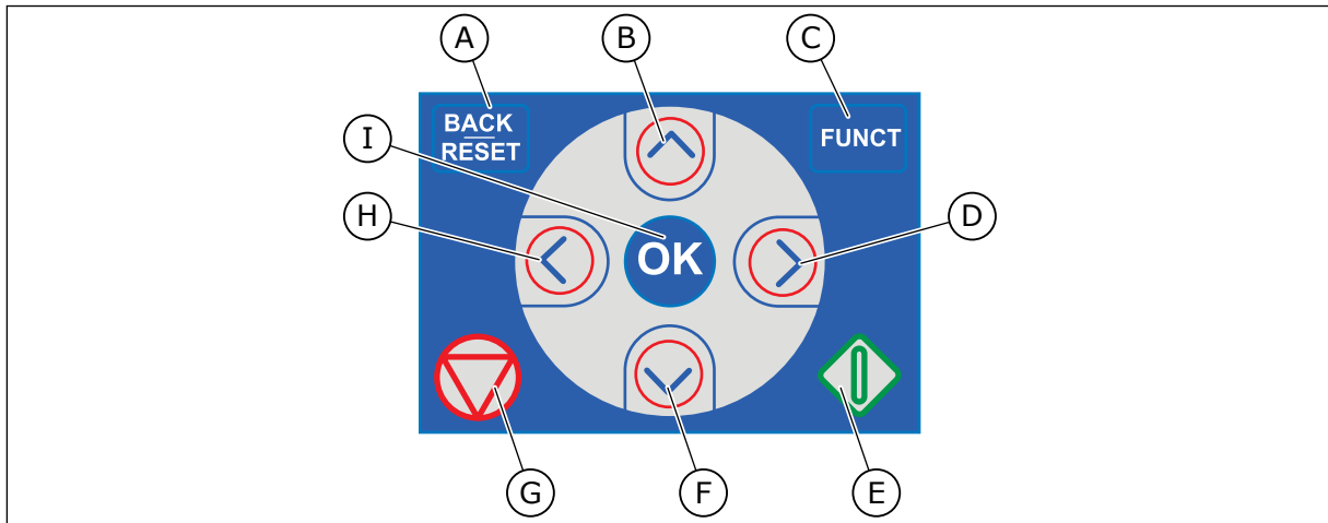
Рис. 1: Кнопки клавиатуры
