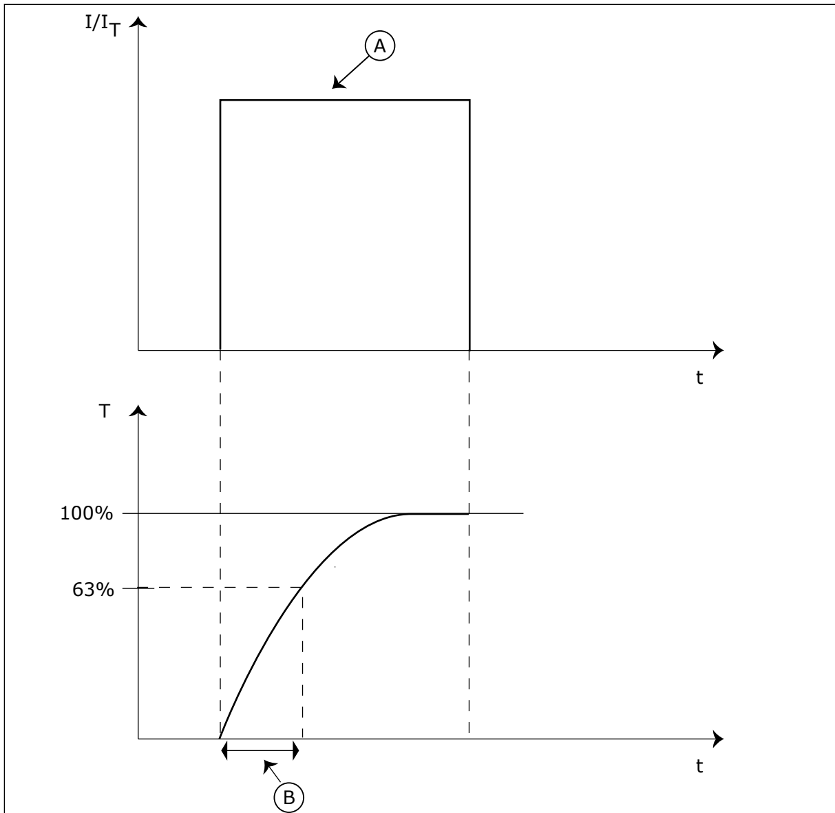
Рис. 66: Тепловая постоянная времени двигателя
