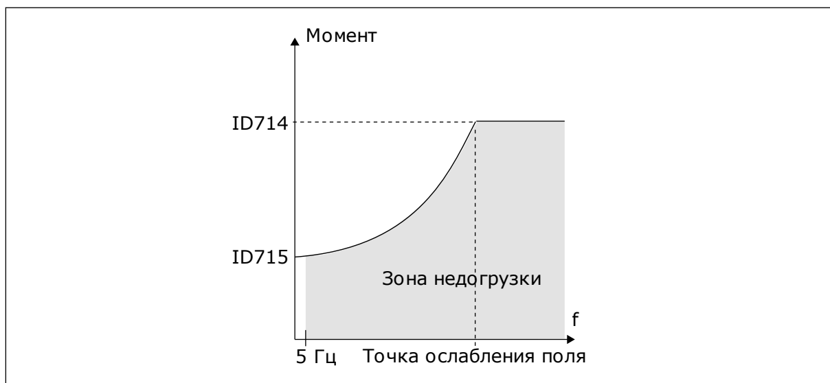
Рис. 69: Настройка минимальной нагрузки
