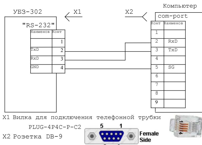
Рисунок 2.2 - Схема подключения УБЗ-302 к компьютеру
