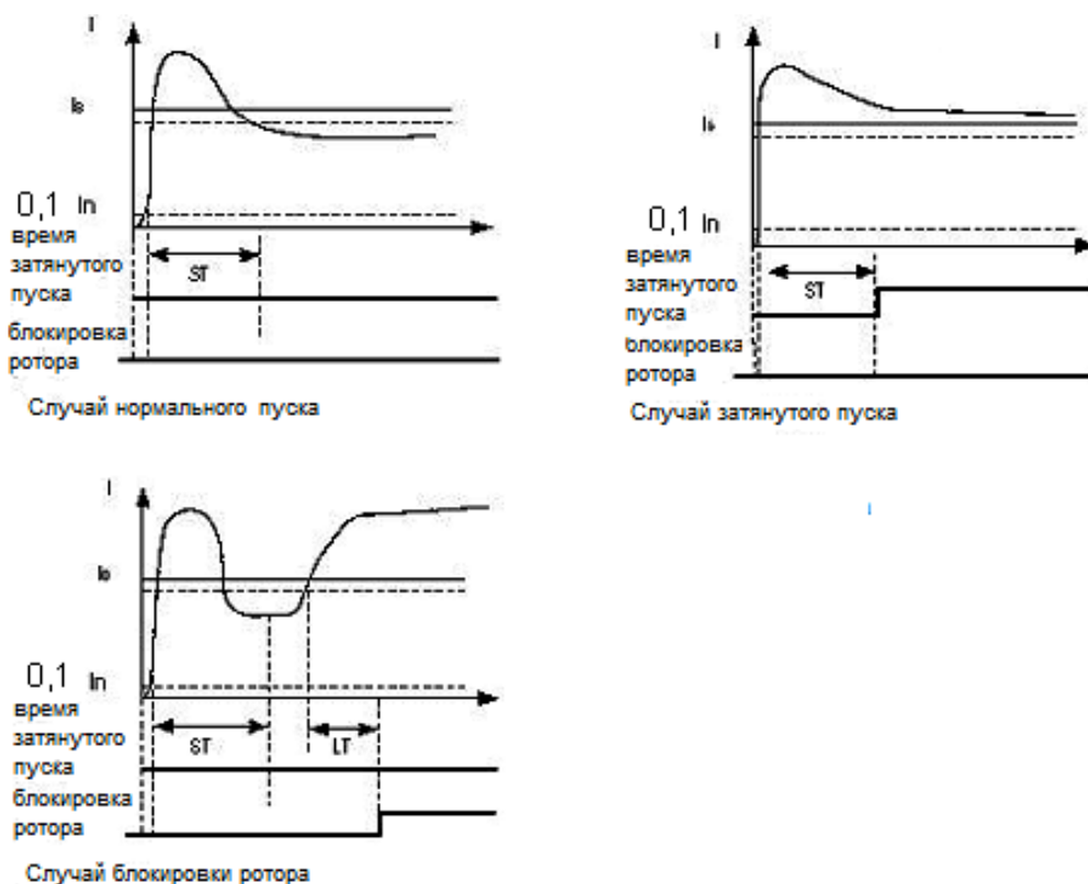
Рисунок 1.4 - Затянутый пуск и блокировка ротора
