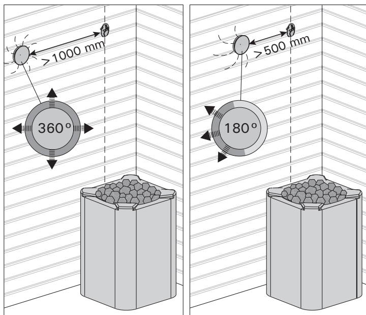
Kuva 11. Anturin minimiet isyys tuloilmaventtiilistä
