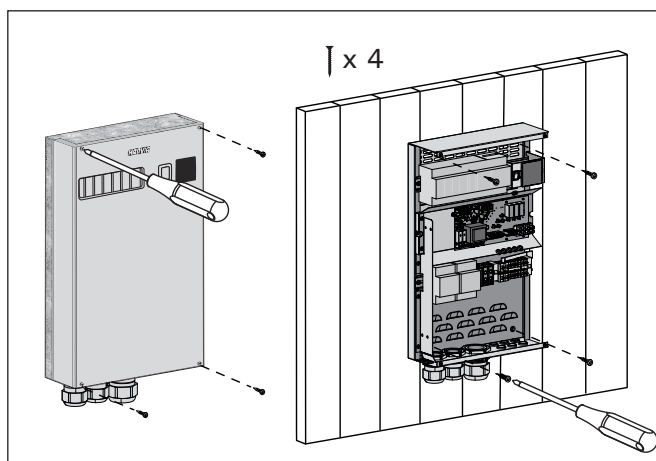
Kuva 7. Ohjauskeskuksen kannen avaaminen ja kiinnittämisen seinään
