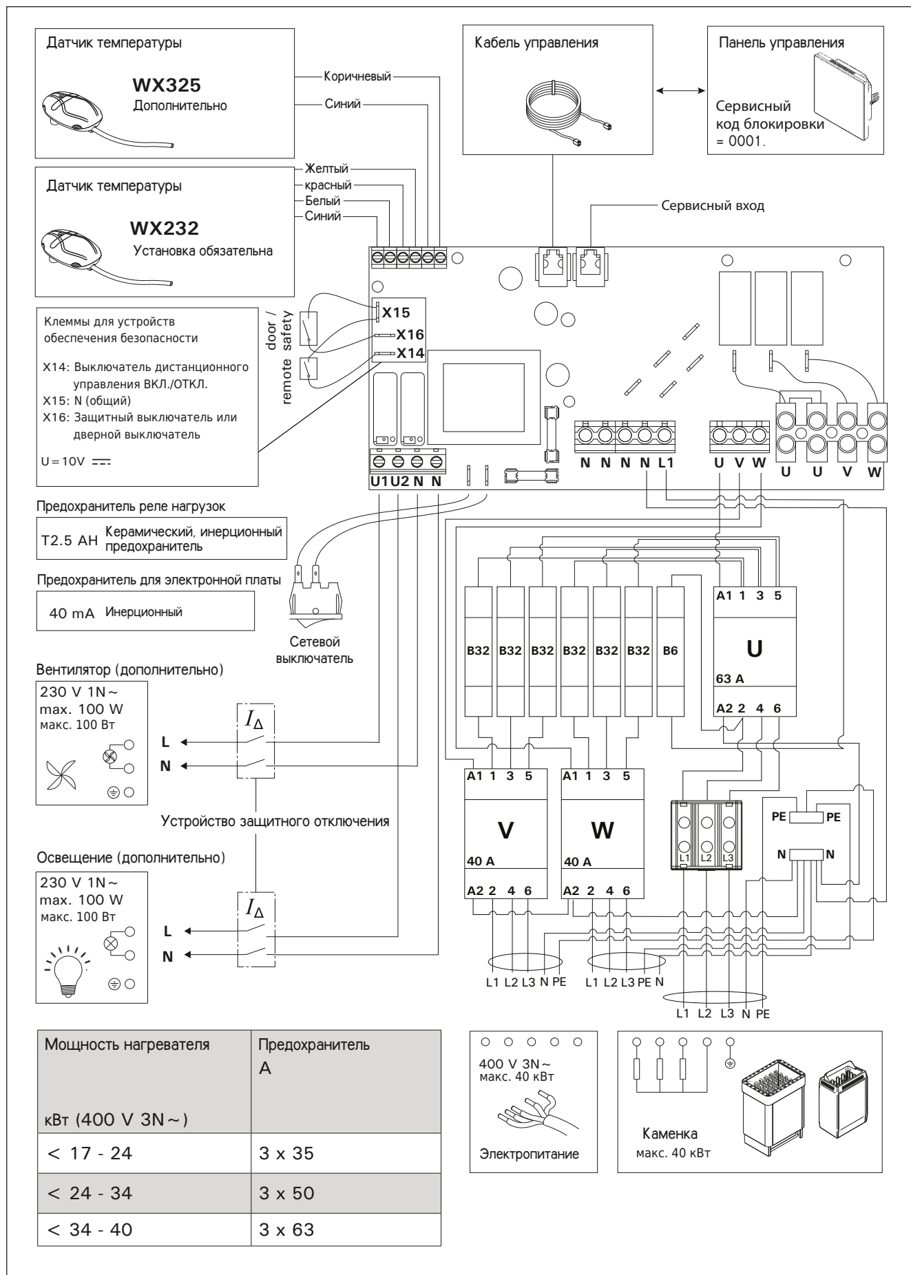
Рис. 8. Электрические подключения
