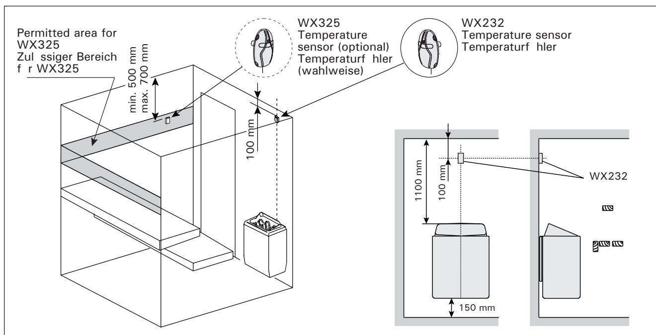
Figure 9. The place of the temperature sensors in connection with wall-mounted heaters Abbildung 9. Position der Temperatursensoren bei Saunen mit Wandbefestigung
