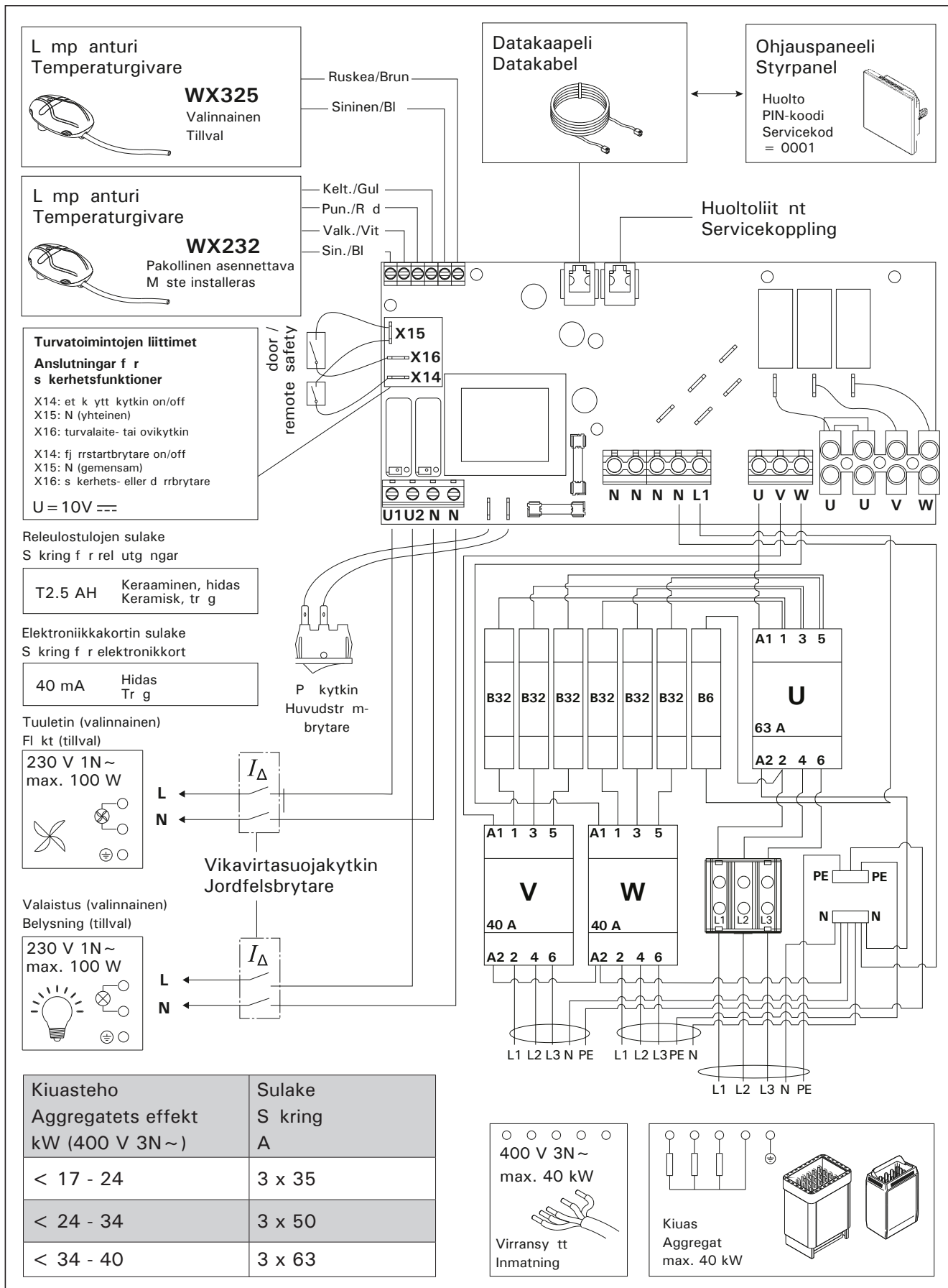
Kuva 8. Sähkökytkennät Bild 8. Elektriska anslutningar
