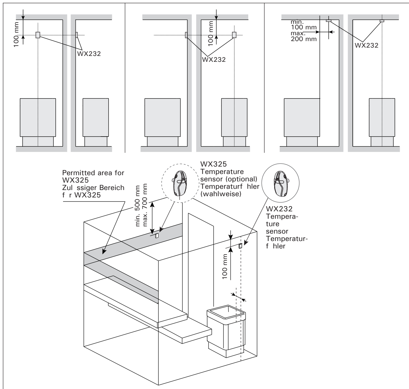
Figure 10. The place of the temperature sensors in connection with floor-mounted heaters Abbildung 10. Position der Temperaturfühler bei Freistehende fen
