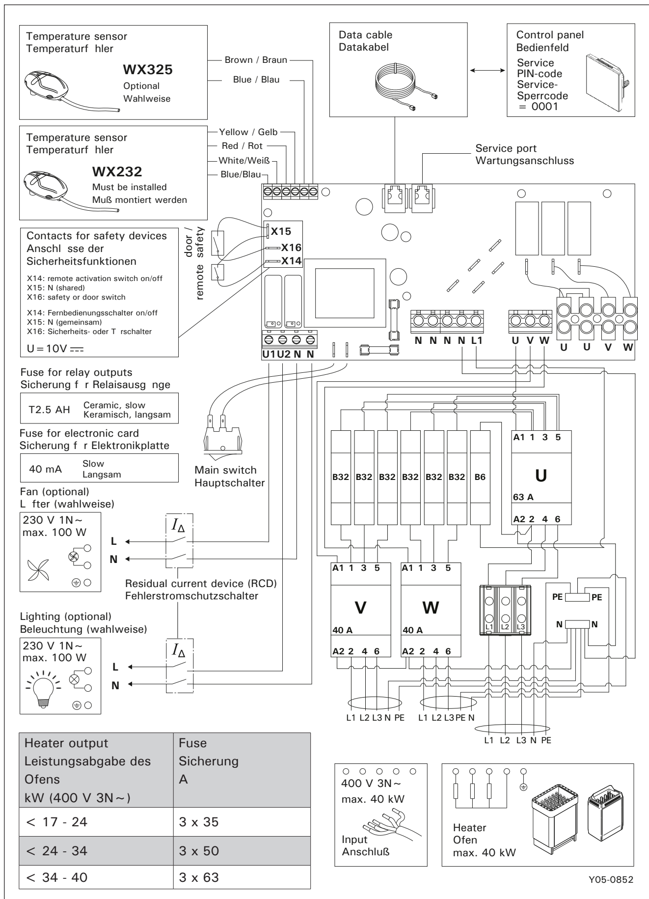
Figure 8. Electrical connections Abbildung 8. Elektrische Anschlüsse
