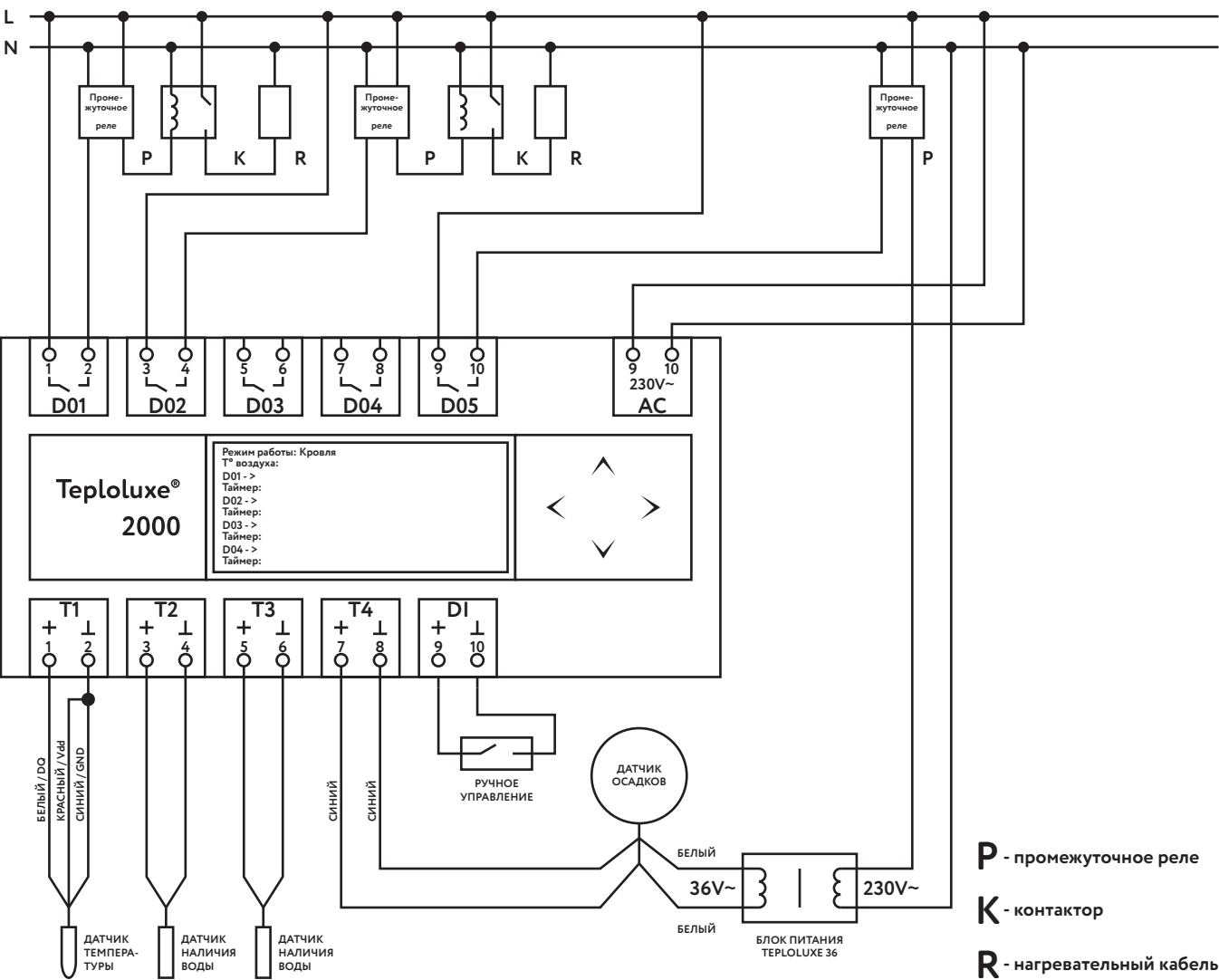
Рис. 3.1.1. Принципиальная схема подключения в режиме «Кровля»
