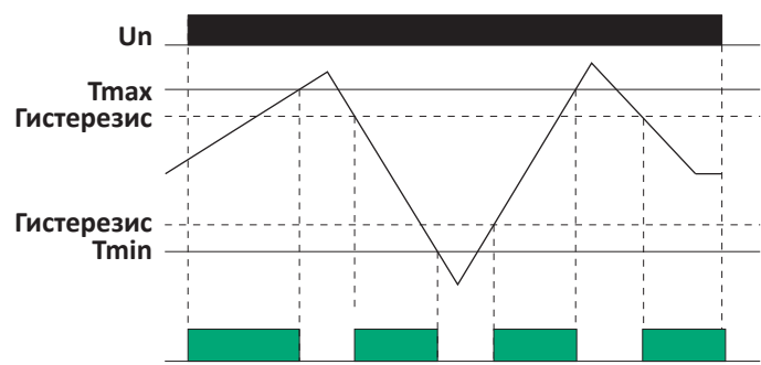
Рис. 3.2.4. Принцип работы гистерезиса DO1
