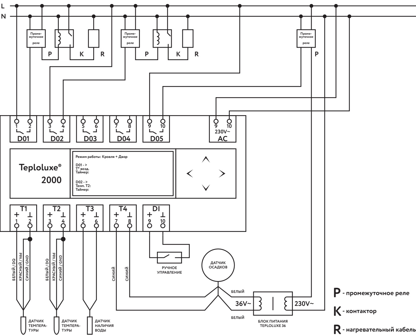
Рис. 3.2.1. Принципиальная схема подключения в режиме «Кровля + Двор»
