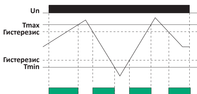
Рис. 3.1.3. Принцип работы гистерезиса
