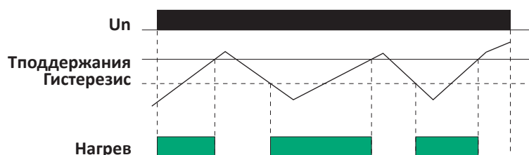
Рис. 3.3.3. Принцип работы гистерезиса канала DO1 и DO2
