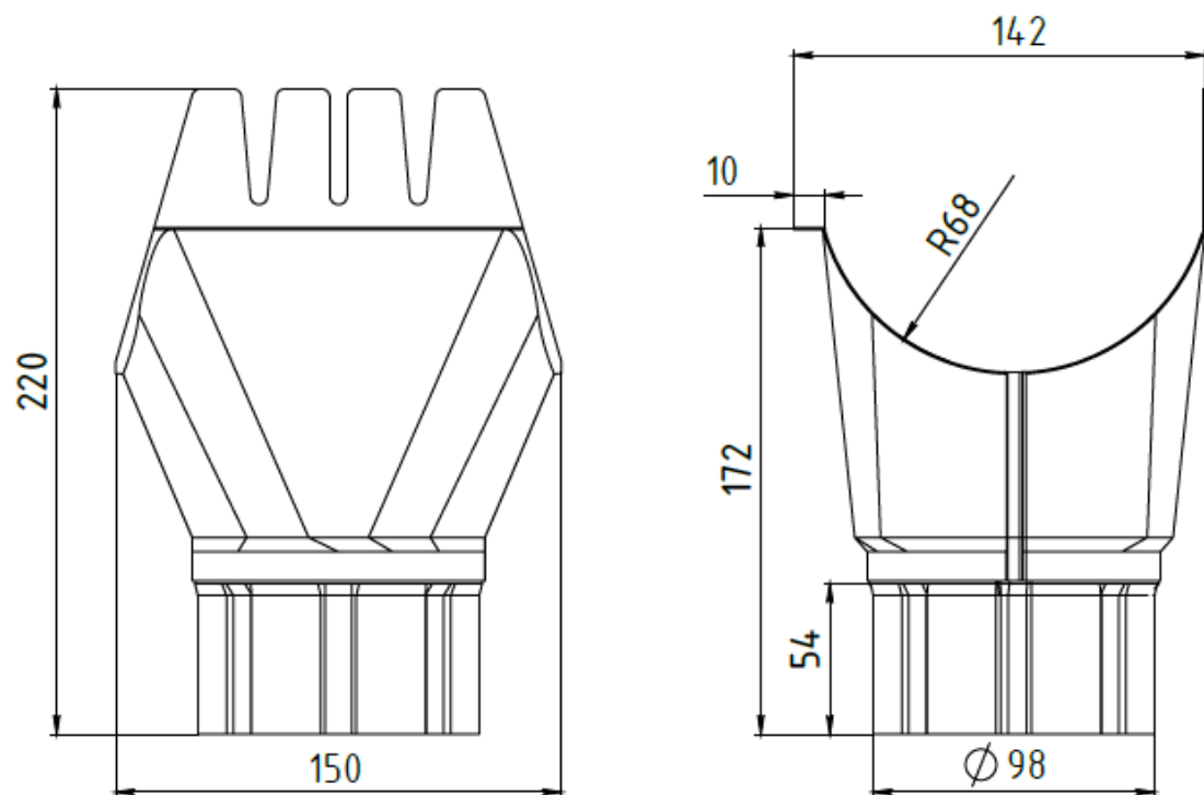
Чертеж Воронка выпускная 125x100 мм
