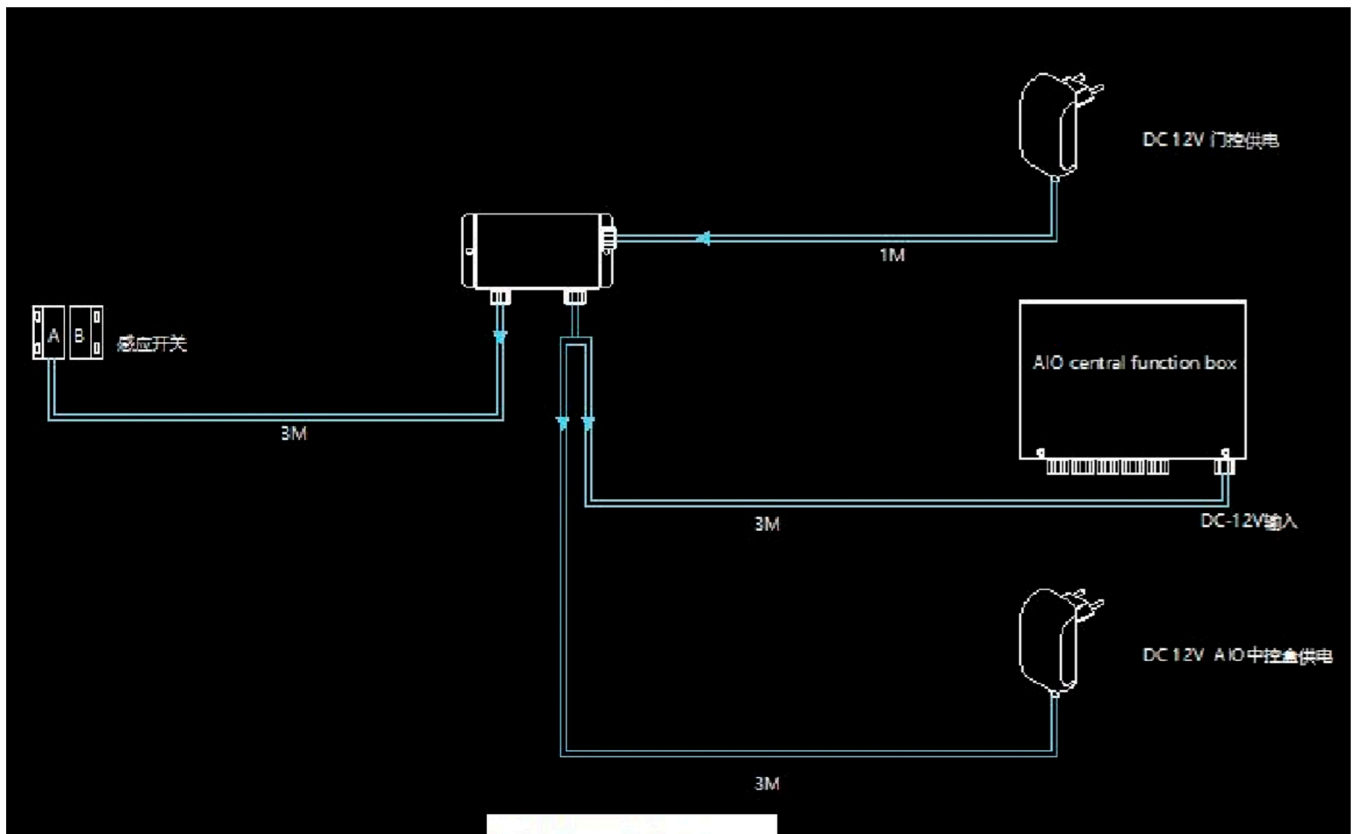
Схема подключения:
