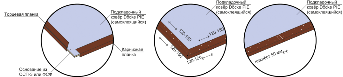
Рис. 13. Крепление металлических карнизных и торцевых планок.
