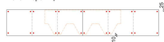
Рис. 17. Схема крепления коньково-карнизной черепицы Döcke на карнизе.
