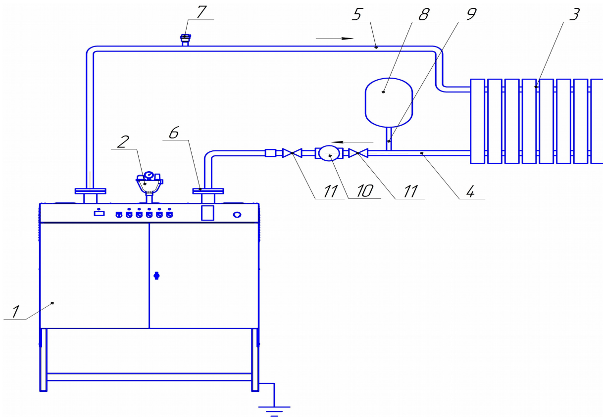
4-сур. Жылыту жүйесінде ЭВН-К пайдалану нұсқасы
