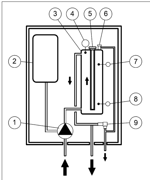
Рисунок 1. Принципиальная схема котла
