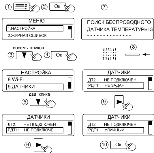
Рисунок 24. Настройка радиодатчиков
