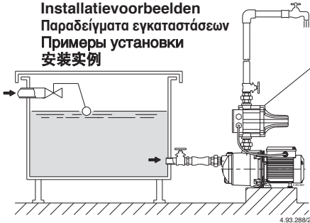
Fig. 2 Funzionamento sotto battente Positive suction head operation Zulaufbetrieb Fonctionnement en charge Funcionamiento bajo carga Tillrinning sugsidan Toelooisituatie Θέση λειτουργίας με θετική αναρρόφηση Работа под гидравлическим давлением 入口正压头
