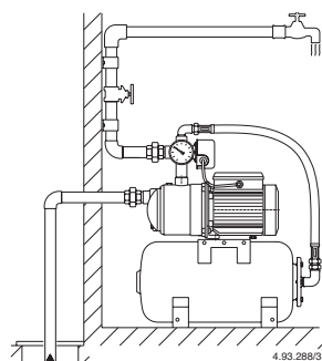
Fig. 2 Funzionamento in aspirazione Suction lift operation Saugbetrieb Fonctionnement en aspiration Funcionamiento en aspiración Sugande funktion Zuigsituatie Θέση λειτουργίας με κάθete αναρρόφηση Работа выше уровня жидкости 负压水头工作
