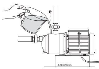
Fig. 4 Riempimento Filling Auffüllung Remplissage Llenado Fyllning Vullen Γέμισμα Наполнение 灌泵
