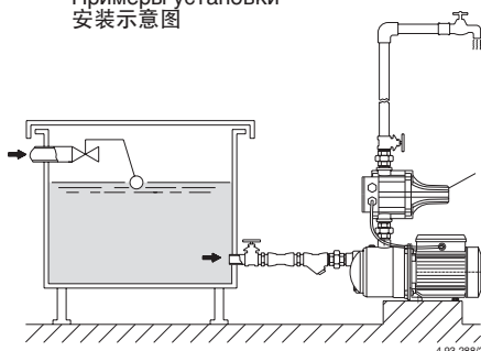
Fig. 1 Funzionamento sotto battente Positive suction head operation Zulaufbetrieb Fonctionnement en charge Funcionamiento bajo carga Tillrinning sugsdan Toeloopsituatie Θέση λειτουργίας με θετική αναρρόφηση Работа под гидравлическим напором 正压上水头的操作
