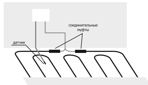
Рисунок 4. Установка датчика в стяжке пола
