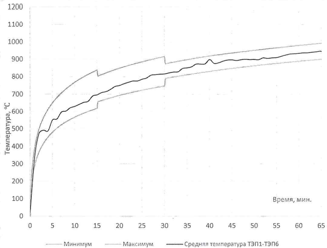
Рис. 5. Изменение температурного режима в огневой камере печи. Образец № 2.
