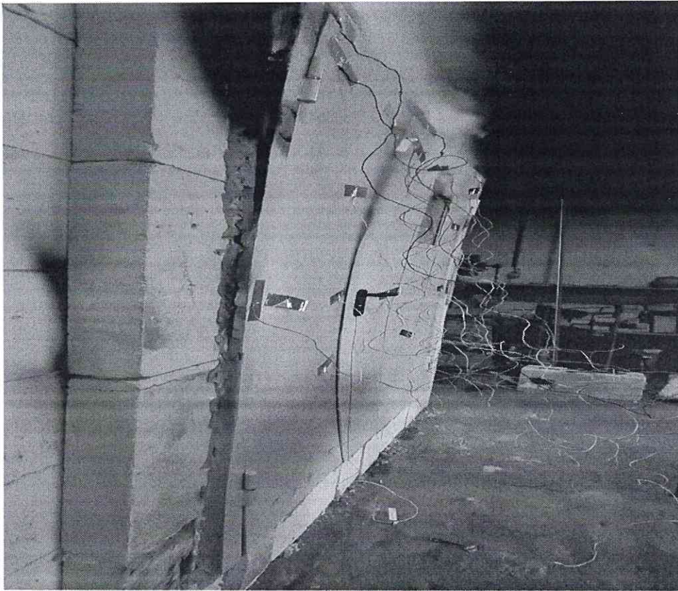
Вид образца во время проведения испытаний
