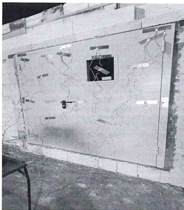
Вид образца до проведения испытаний
