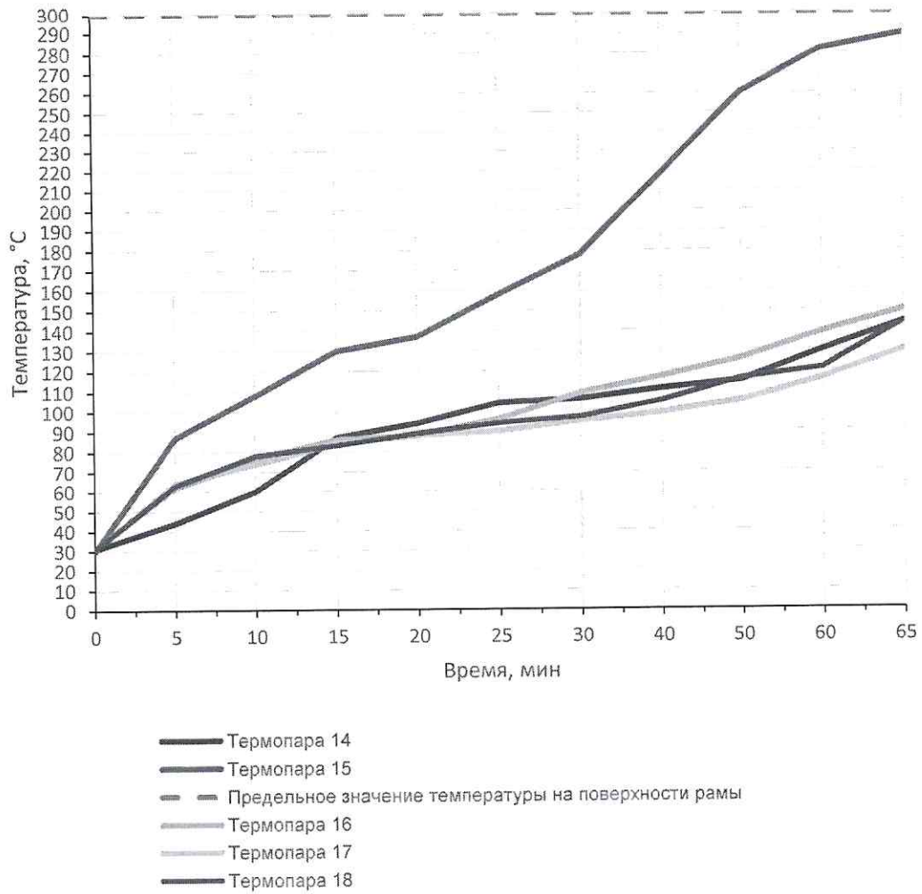
Рис. 8. Изменения температуры на необогреваемой поверхности коробки образца № 1.
