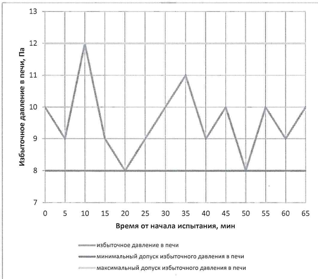
Рис. 6. Изменение избыточного давления в печи. Образец № 2.
