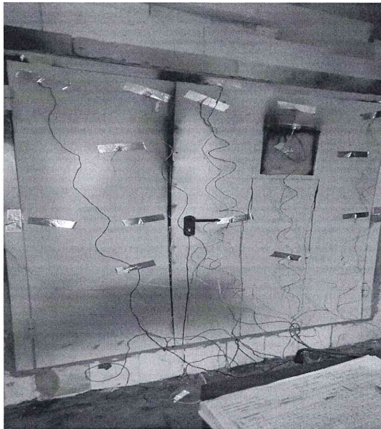
Вид образца во время проведения испытаний
