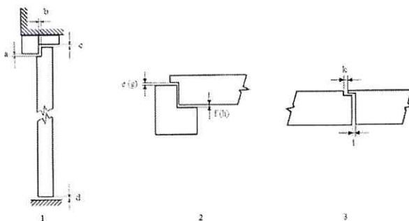
Рис. 1. Схема измерения зазоров на опытном образце: верхней и нижней стороне – 1, на боковых сторонах – 2, между полотнами – 3.
