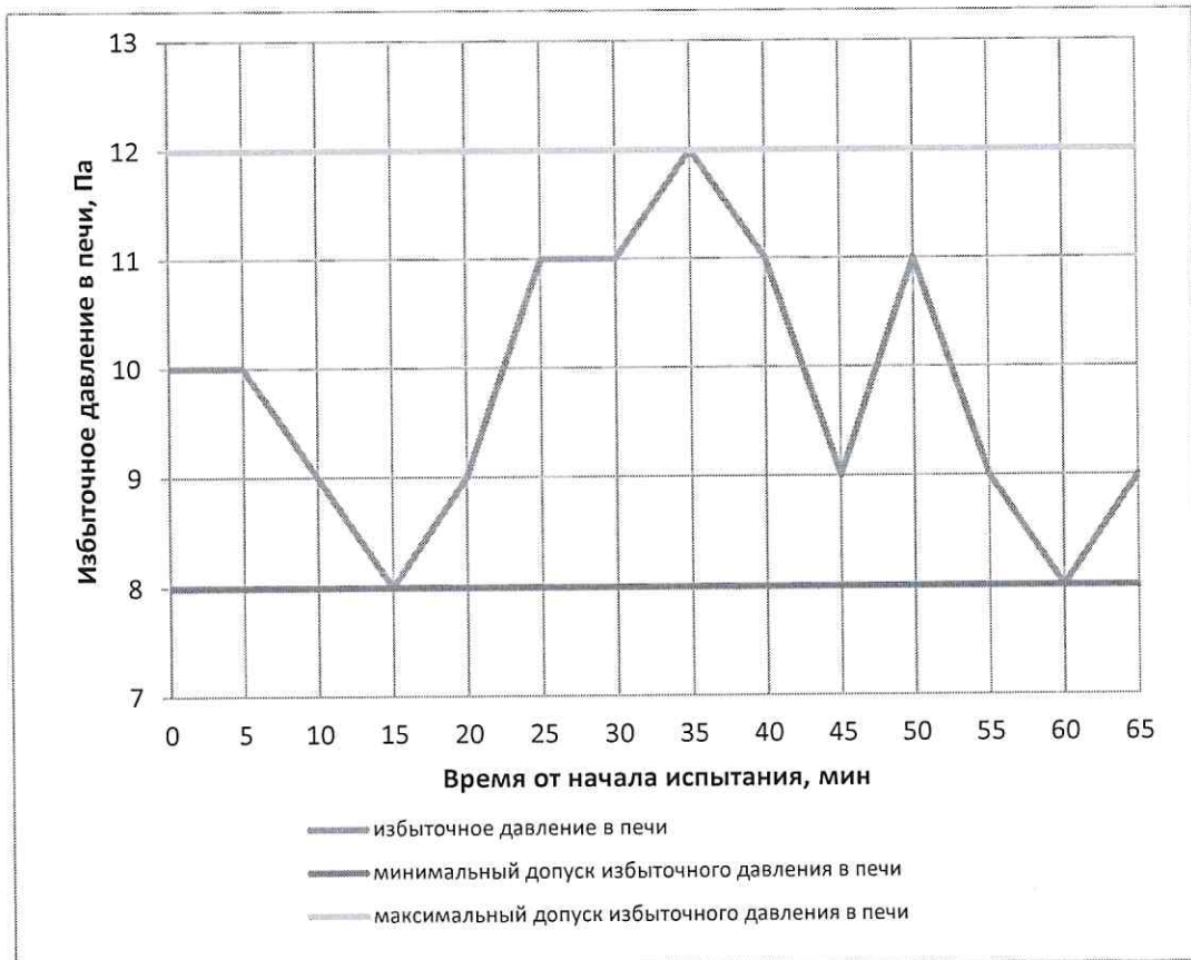
Рис. 4. Изменение избыточного давления в печи. Образец № 1.
