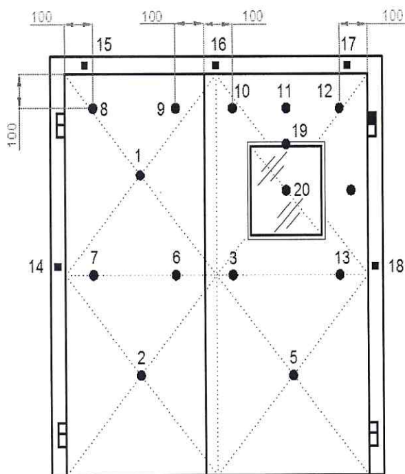
Рис. 2. Схема расстановки термомпар.
