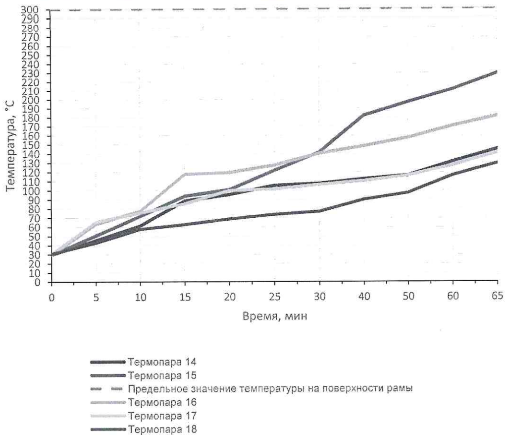
Рис. 10. Изменения температуры на необогреваемой поверхности коробки образца № 2.
