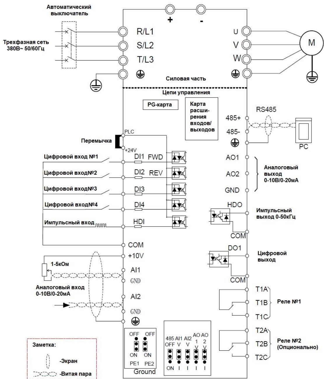
Рисунок 2 – Схема подключений для VFD500-630GT4
