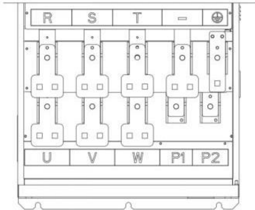
Рисунок 3 – Вид силовых клемм для VFD500-630GT4
