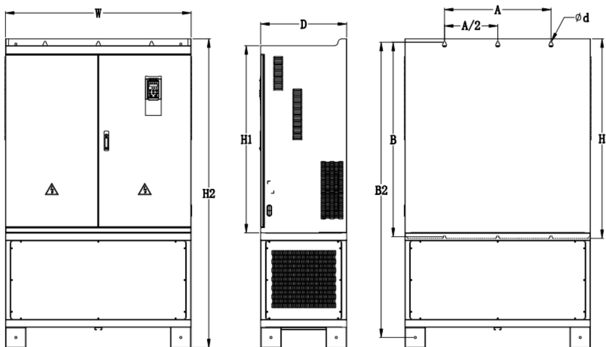
Рисунок 1 – габариты VFD500-630GT4.
