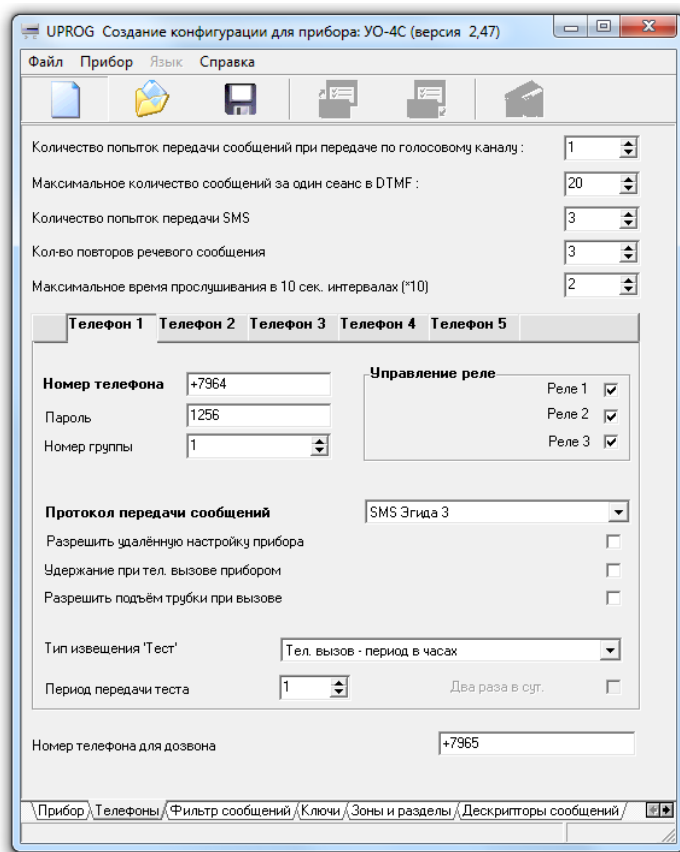
Рисунок 13. «Телефоны»
