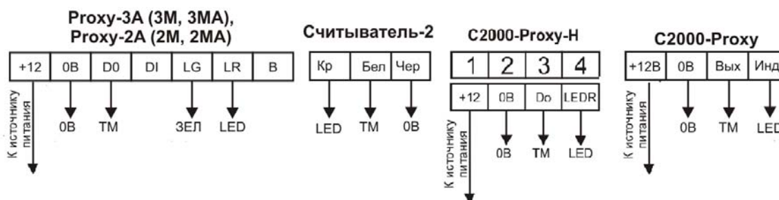
Рисунок 7. Подключение считывателей
