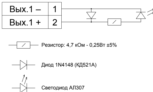
Рисунок 5. Схема имитатора пусковой цепи.
