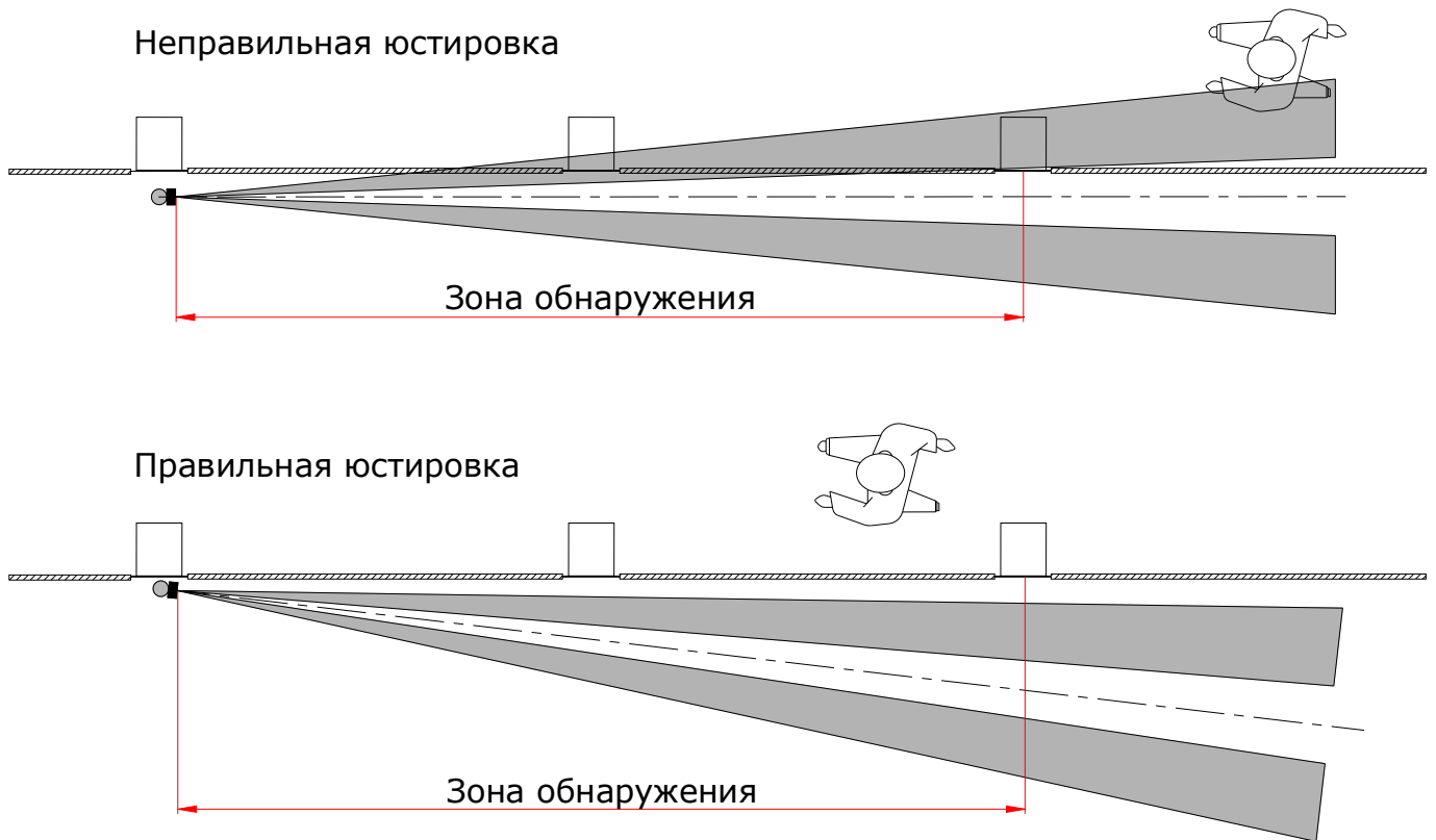
Рис.4 Юстировка извещателя на зону обнаружения.
