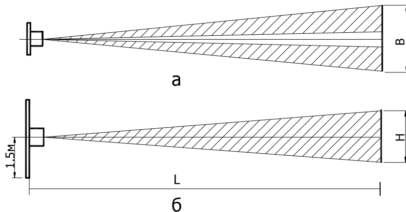
Рис. 1 Диаграмма направленности зоны обнаружения а - охват по горизонтали, б - охват по вертикали; L - длина зоны обнаружения, H - высота, B - ширина.
