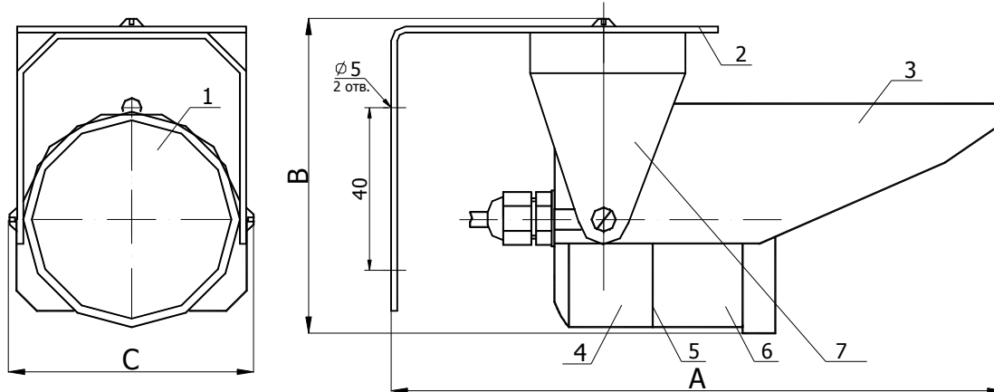
Рис. 2 Общий вид извещателя ИД-40, ИД-50 1-линза френеля, 2-кронштейн, 3-козырек, 4-основание корпуса, 5-уплотнительное кольцо, 6-крышка корпуса, 7-скоба
