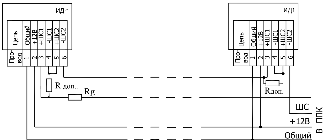
Рис.9 Схема соединения при последовательном включении извещателей на один шлейф. Полярность выходов ШС1, ШС2 условная. Оконечные резисторы R_g на конце шлейфов и R_{доп.} устанавливать в соответствии с документацией на ППК.
