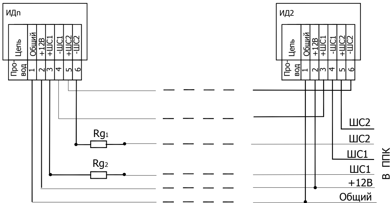
Рис.8 Схема соединения нескольких извещателей с раздельным включением шлейфов.
