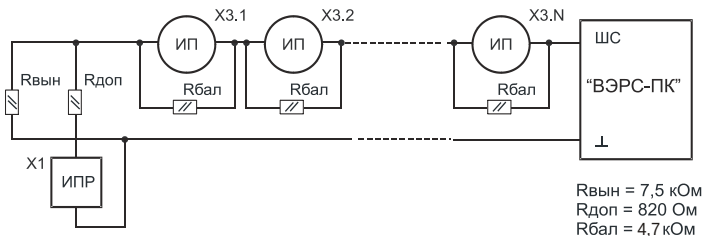
Рис.9. Схемы включения ШС с несколькими тепловыми извещателями (типа ИП-105) и срабаткой по двум извещателям (с перезапросом)
