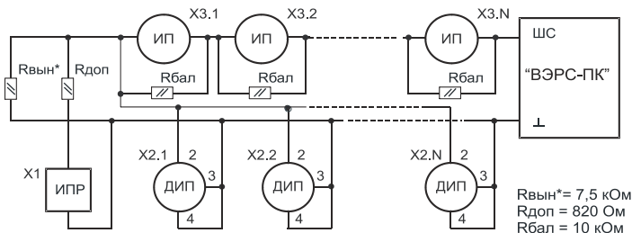
Рис 10. Комбинированная схема включения ШС со срабаткой по одному извещателю (с перезапросом)
