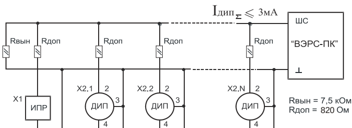
Рис.8 Схемы включения ШС с несколькими дымовыми извещателями (типа ИП212) и срабаткой по двум извещателям (с перезапросом)
