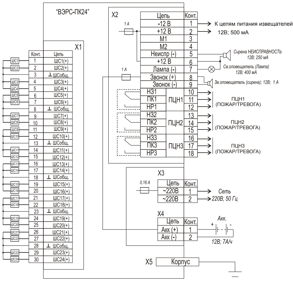
Рис. 7. Схема внешних соединений прибора «ВЭРС-ПК16», «ПК24»
