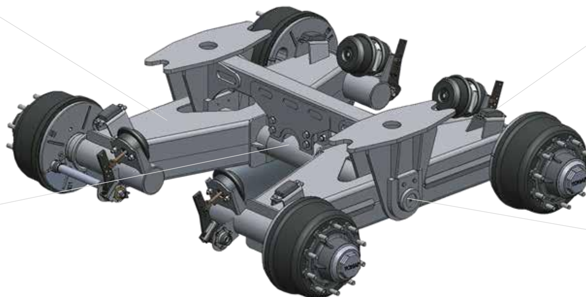
Балансир с полуосями
