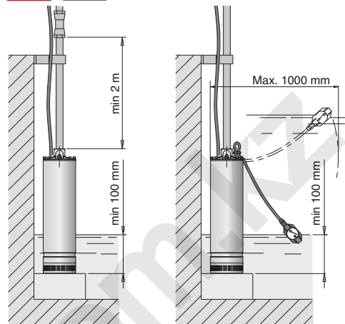
Esecuzione senza galleggianti
