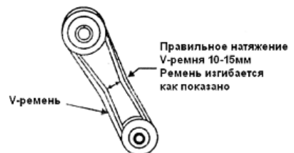
рис. 18 Натяжение V-ремня
