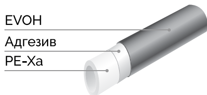
Труба Varmega Flex PE-Xa/EVOH, серая
