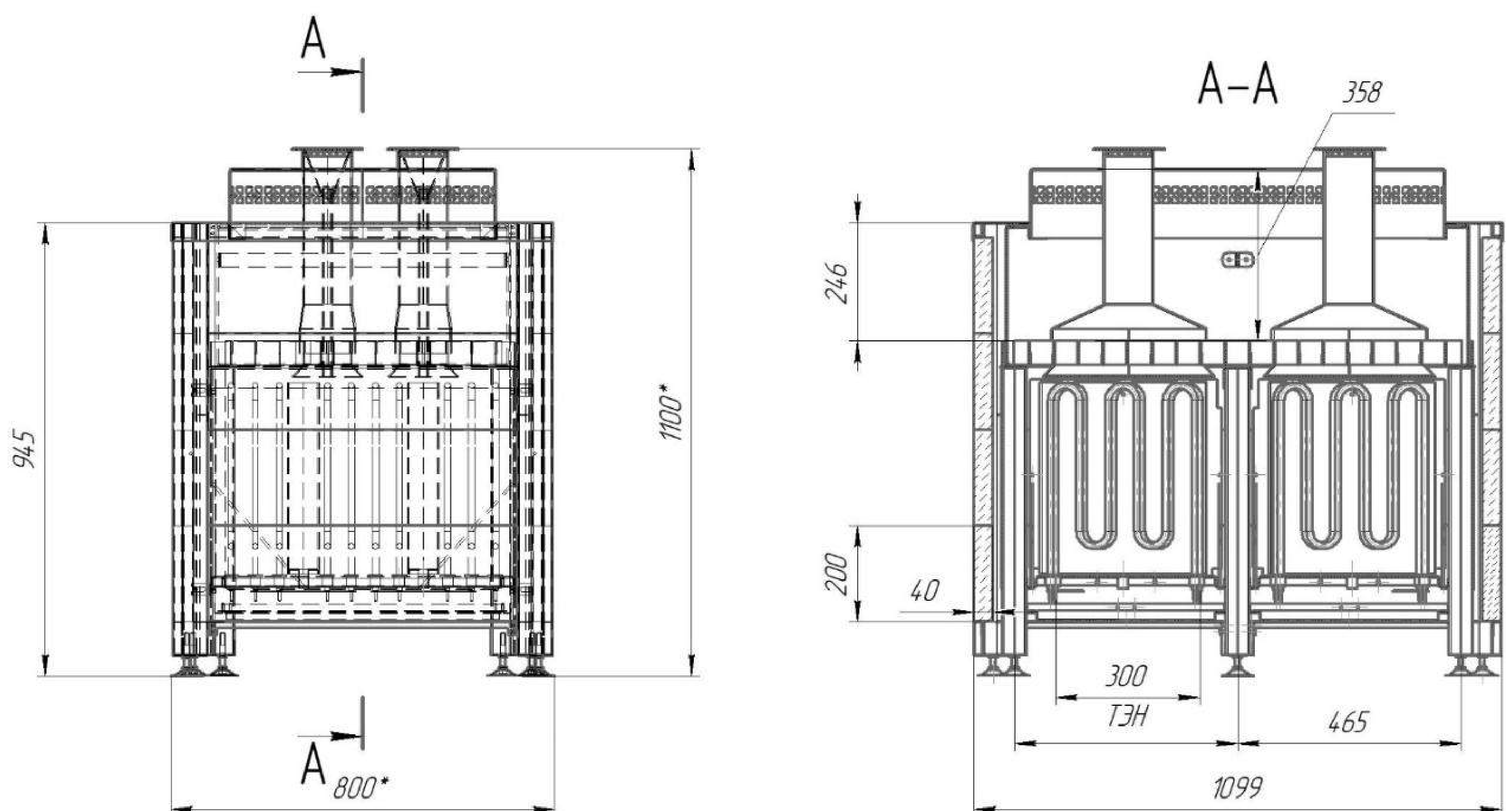
Рис. 1.2.2. Внешний вид Электропечи при двухсекционном исполнении (в разрезе)
