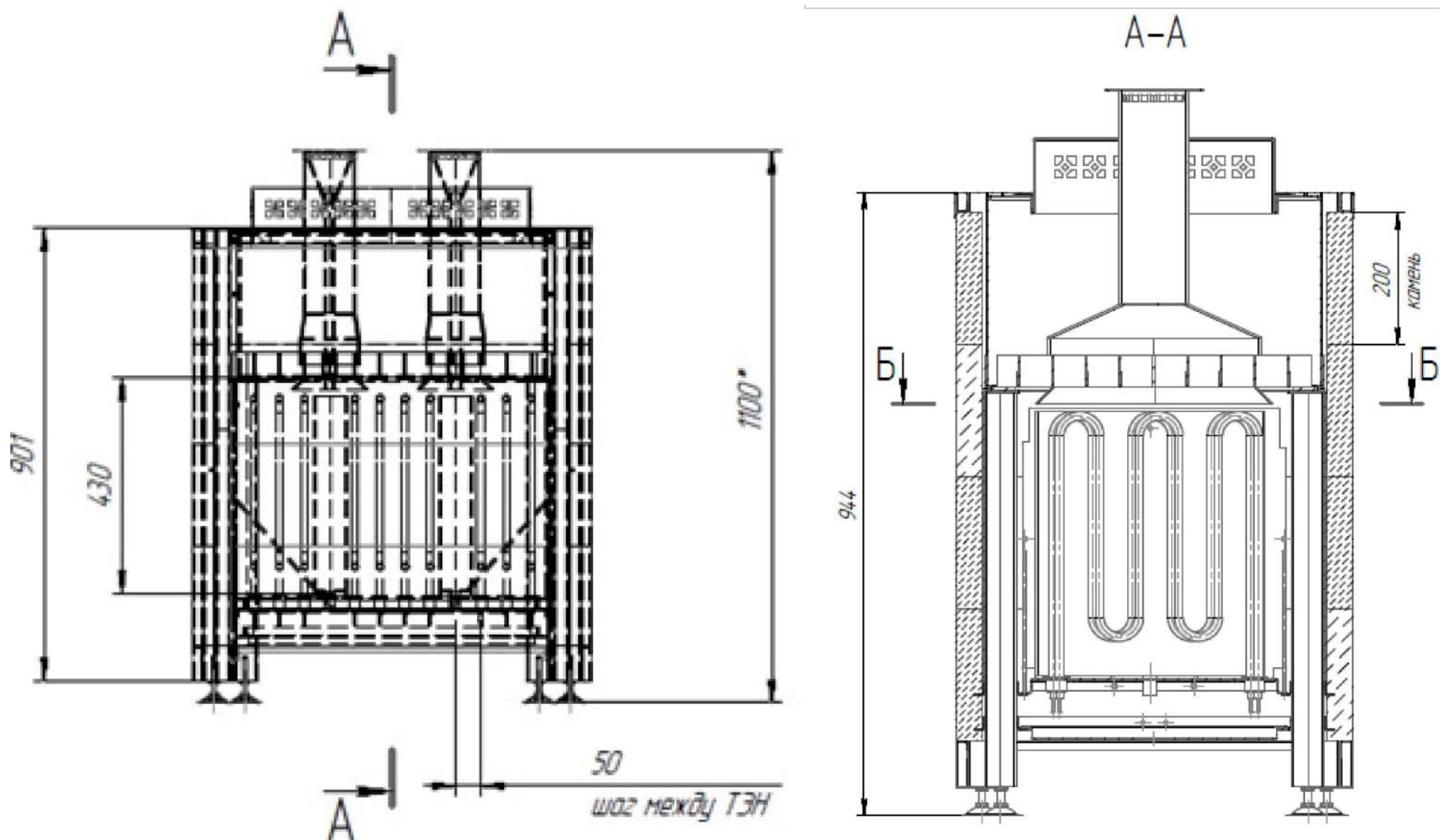
Рис. 1.2.1. Внешний вид Электропечи при односекционном исполнении (в разрезе)
