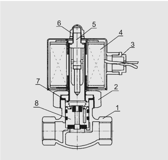
内部结构 Inside Structure
