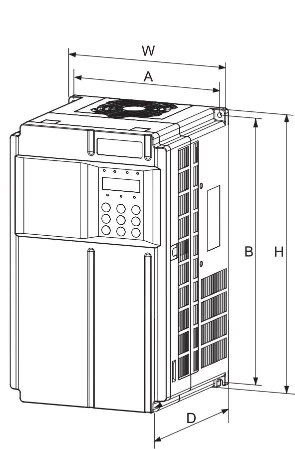
Габаритные и установочные размеры MD290 200G/220P–450G/500P (без дросселя)
